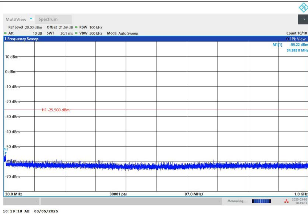
11G-Ant1-2412-30~1000-PASS
