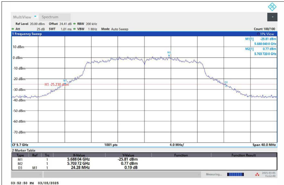
11N20MIMO-Ant2-5700
