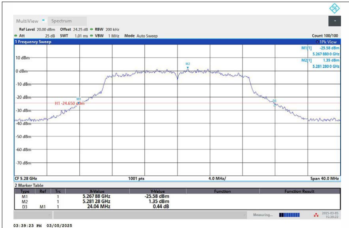
11N20MIMO-Ant2-5280
