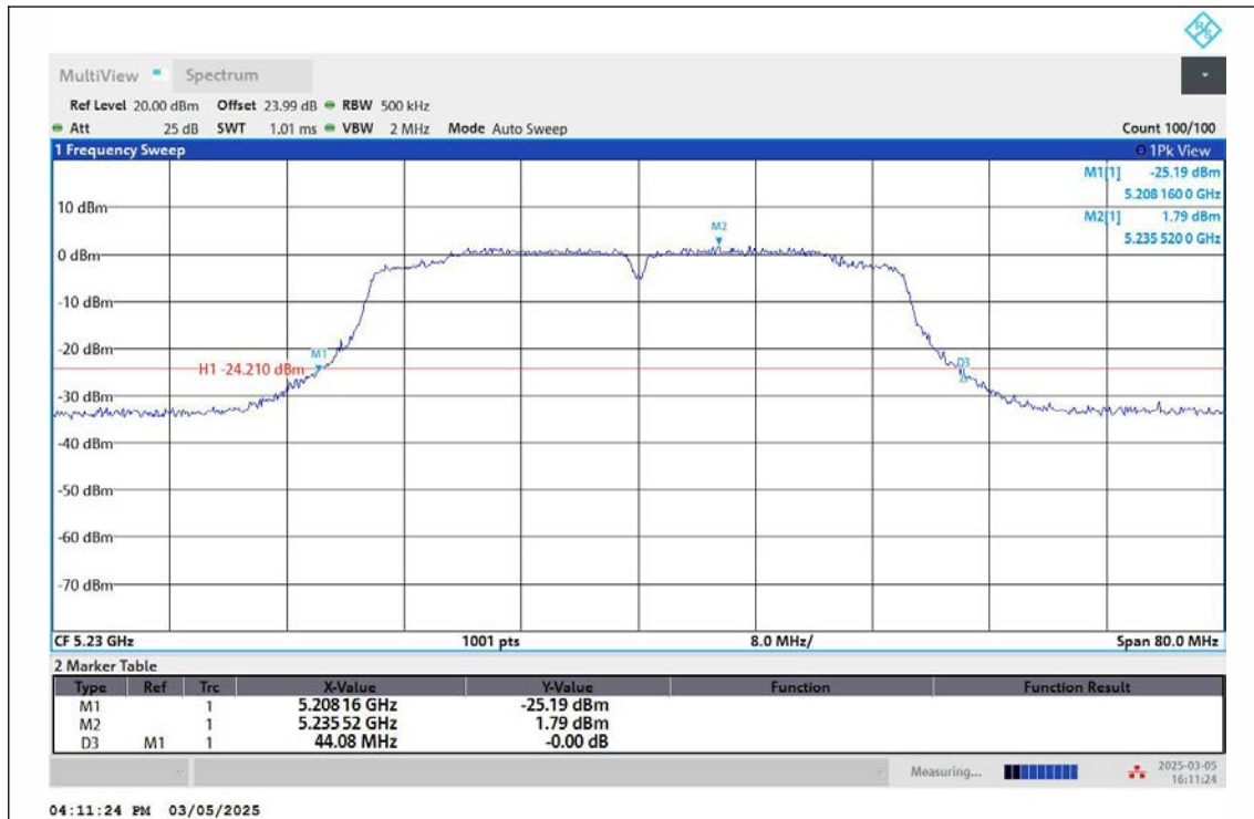
11N40MIMO-Ant2-5230
