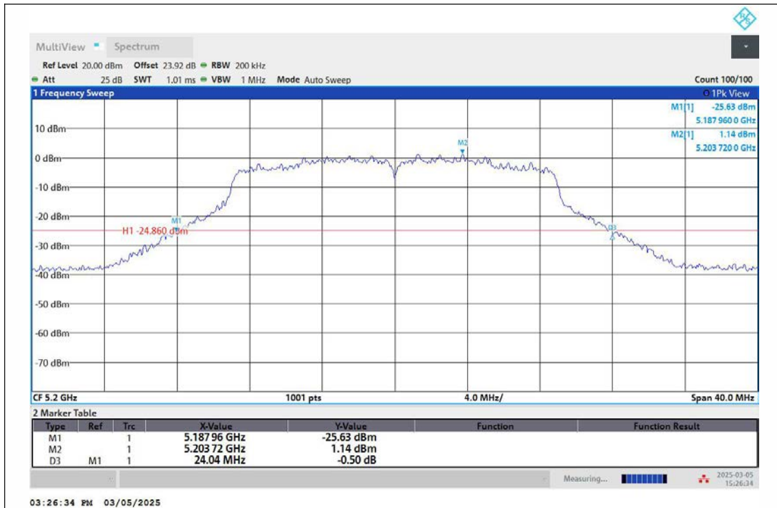
11N20MIMO-Ant2-5200
