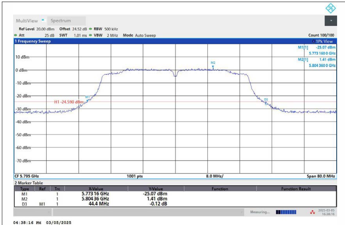
11N40MIMO-Ant2-5795
