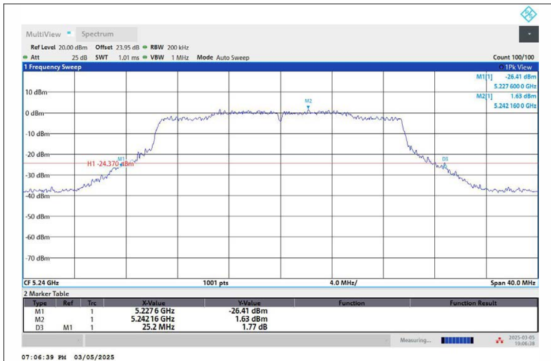
11AX20MIMO-Ant2-5240
