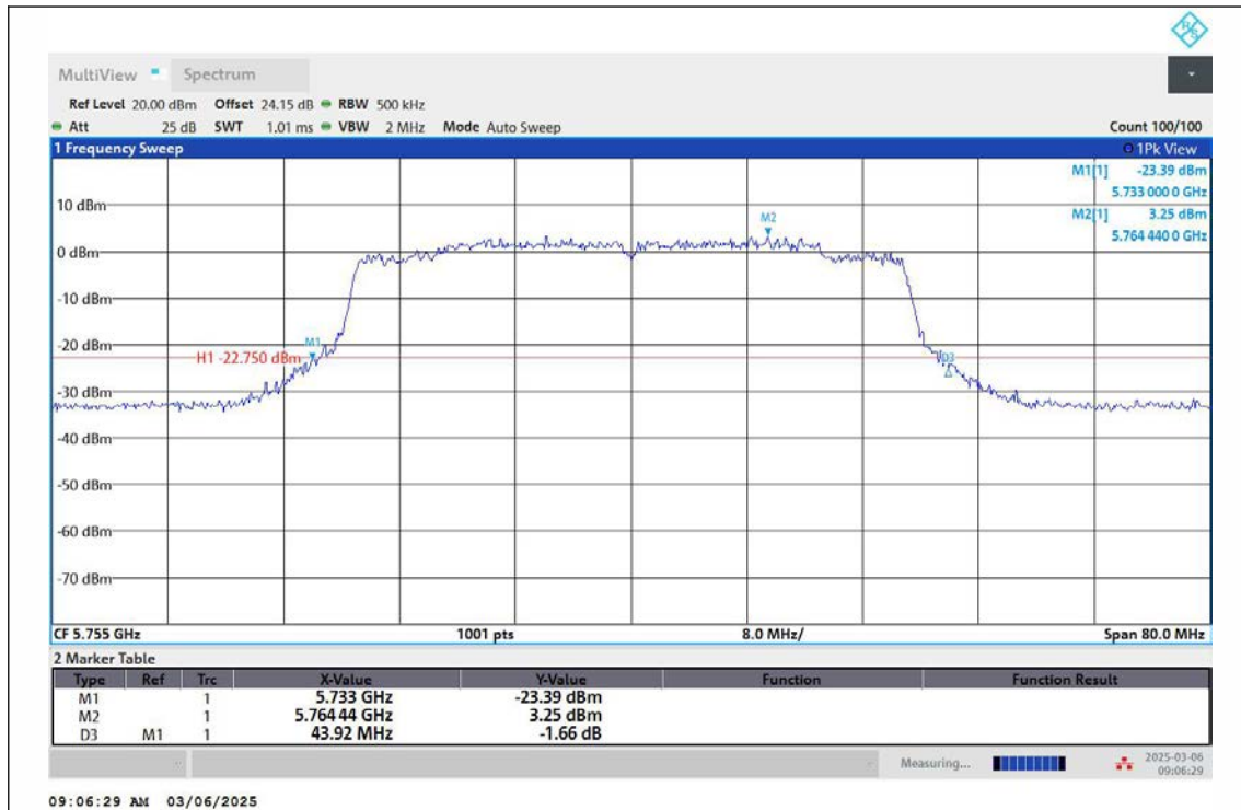
11AX40MIMO-Ant2-5755
