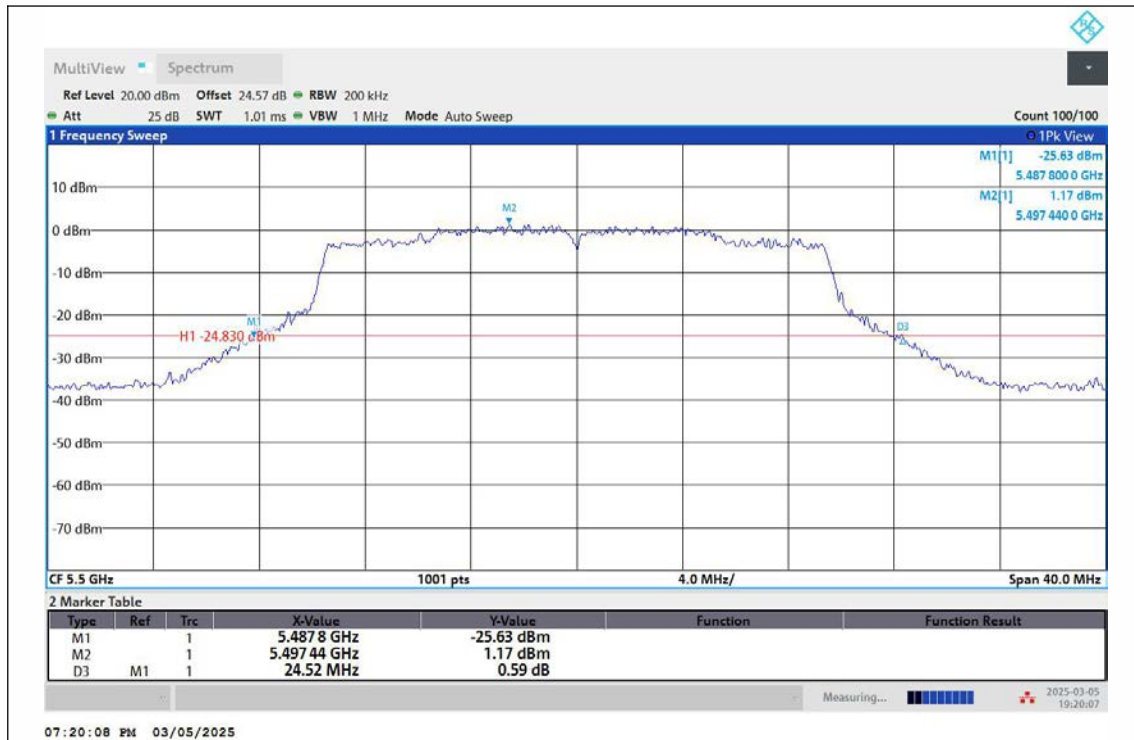
11AX20MIMO-Ant2-5500
