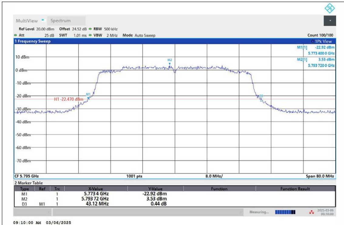
11AX40MIMO-Ant2-5795
