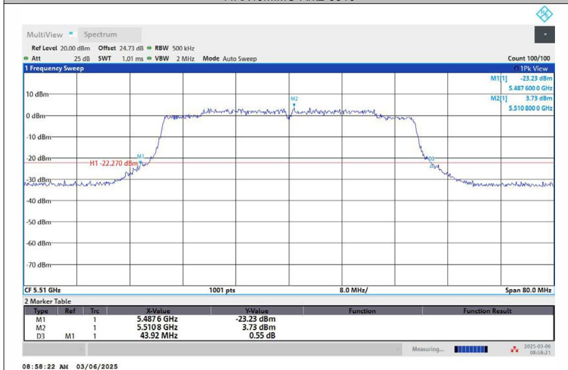
11AX40MIMO-Ant1-5550
