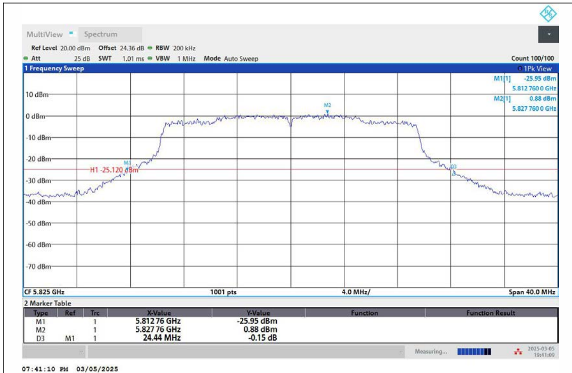
11AX20MIMO-Ant2-5825
