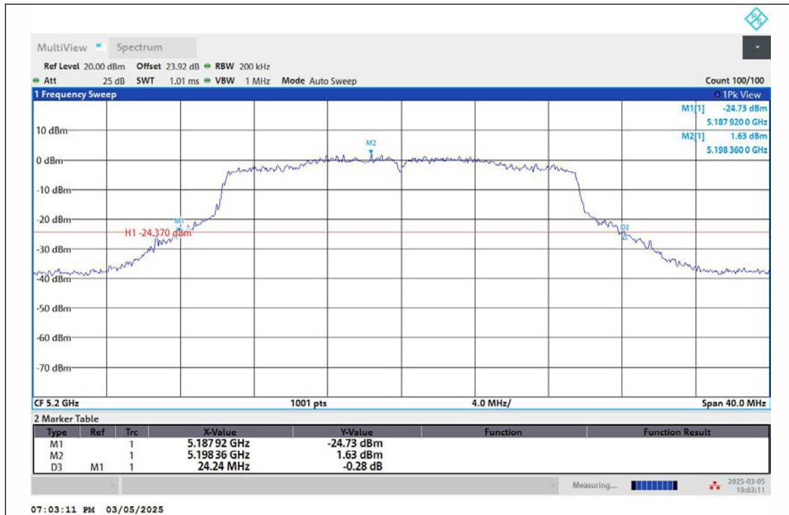
11AX20MIMO-Ant2-5200
