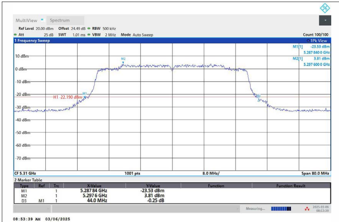
11AX40MIMO-Ant2-5310
