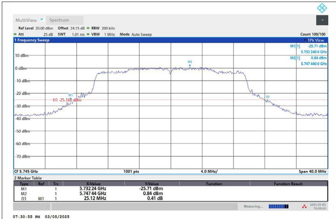
11AX20MIMO-Ant2-5745
