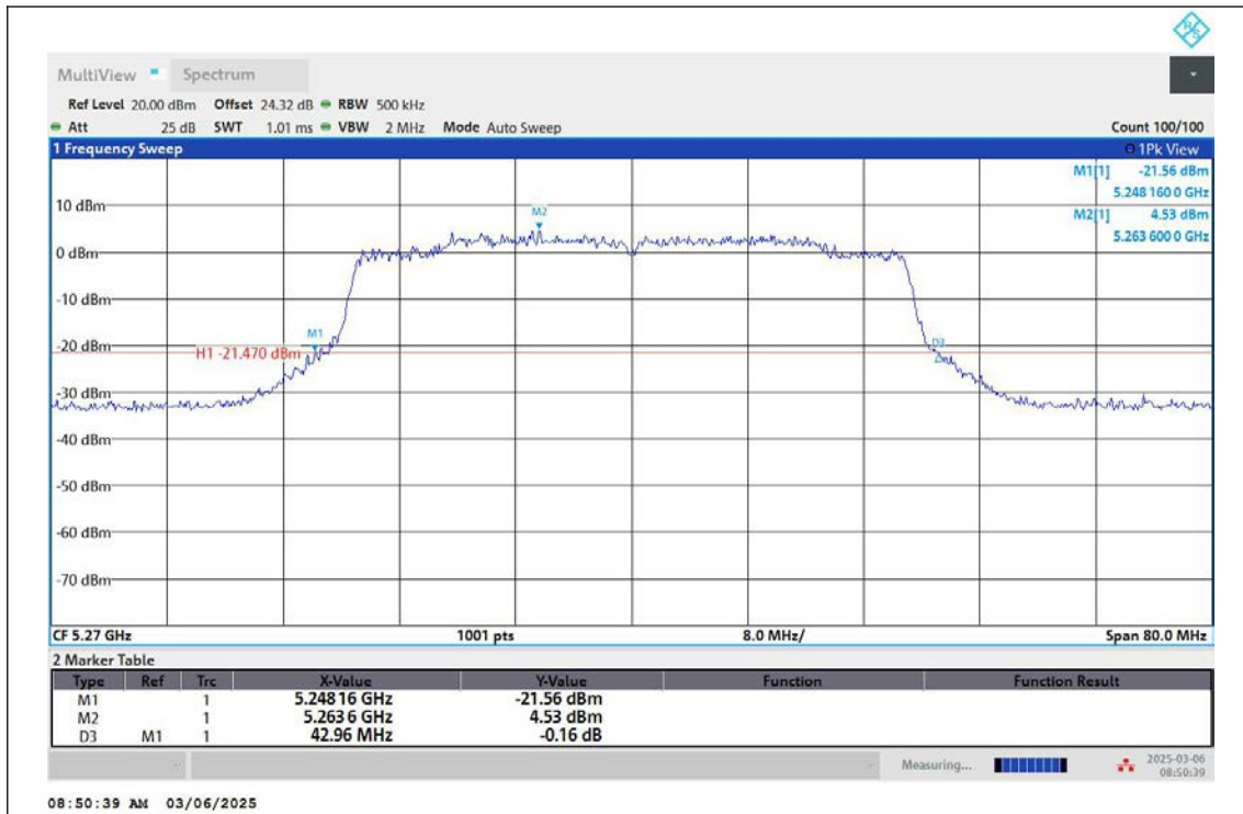
11AX40MIMO-Ant2-5270
