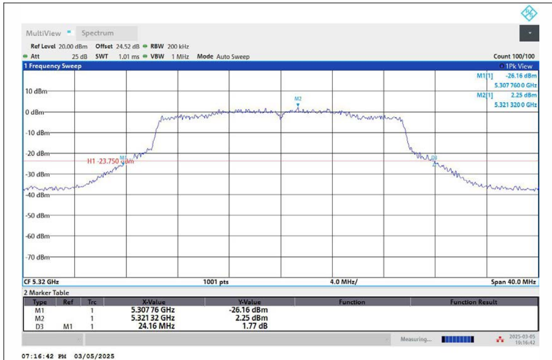
11AX20MIMO-Ant2-5320
