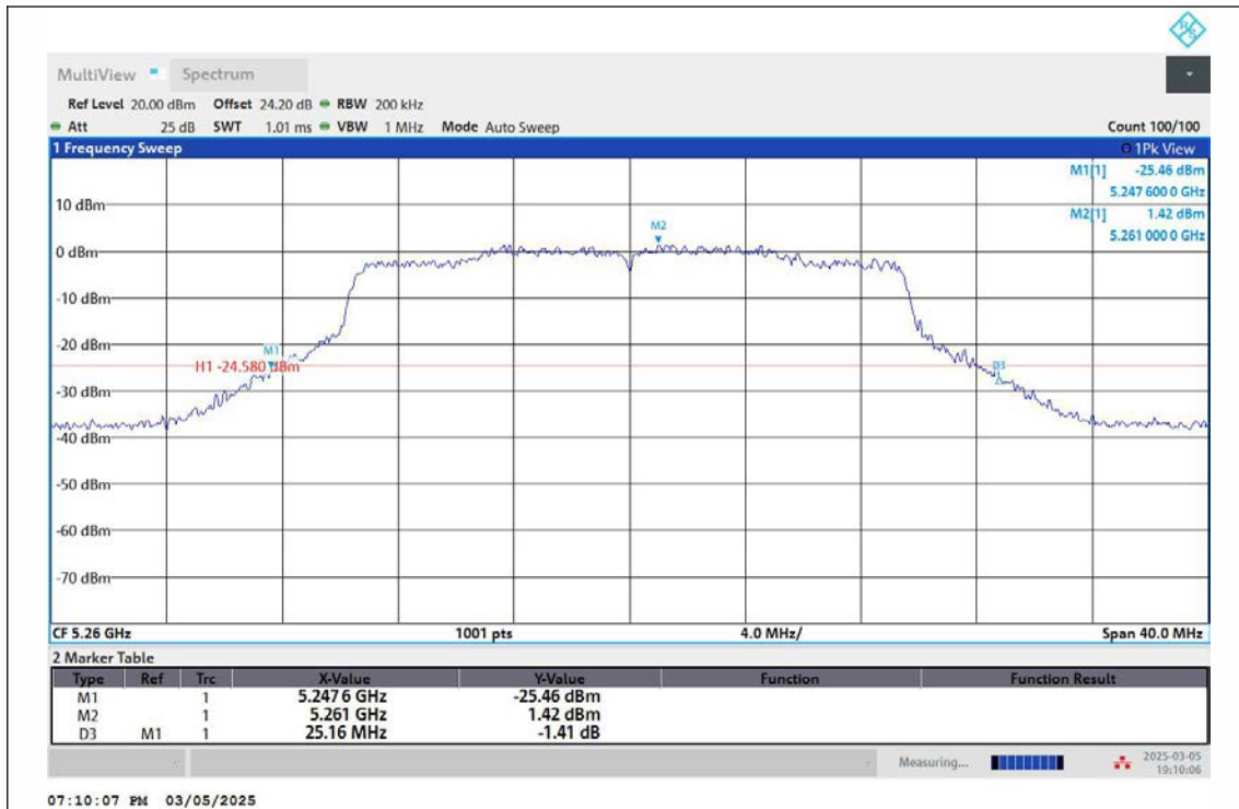
11AX20MIMO-Ant2-5260
