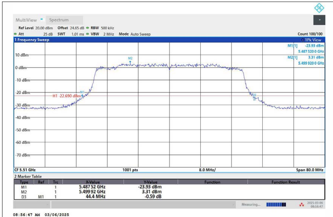
11AX40MIMO-Ant2-5510
