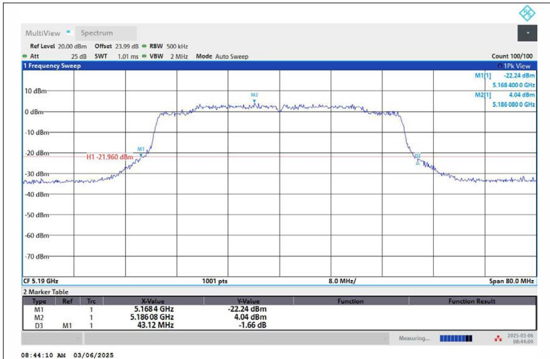
11AX40MIMO-Ant2-5190
