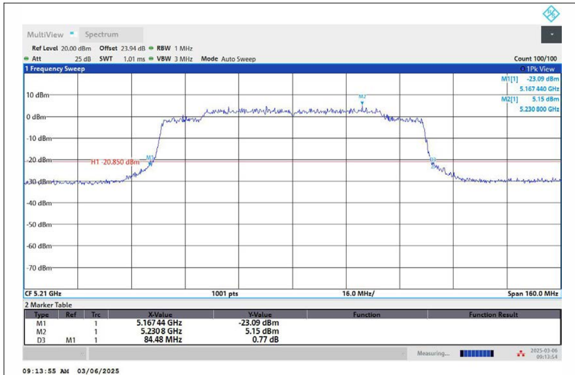
11AX80MIMO-Ant2-5210
