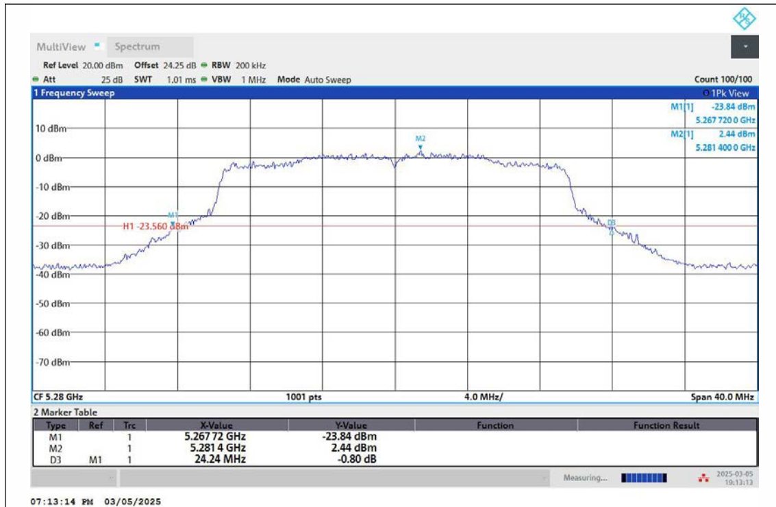
11AX20MIMO-Ant2-5280
