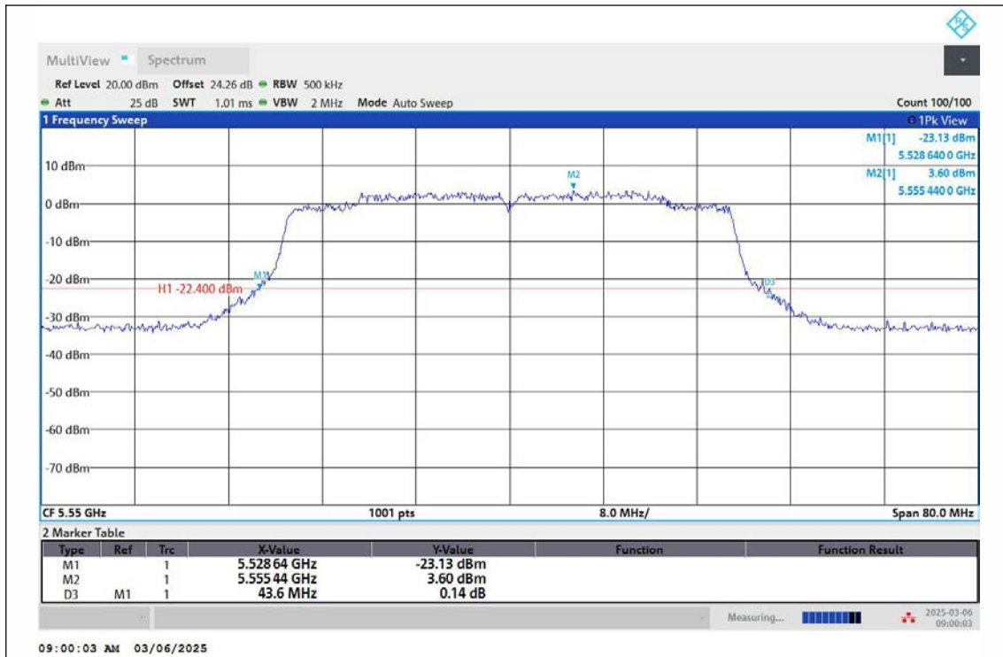
11AX40MIMO-Ant2-5550
