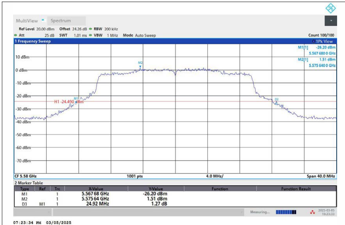
11AX20MIMO-Ant2-5580
