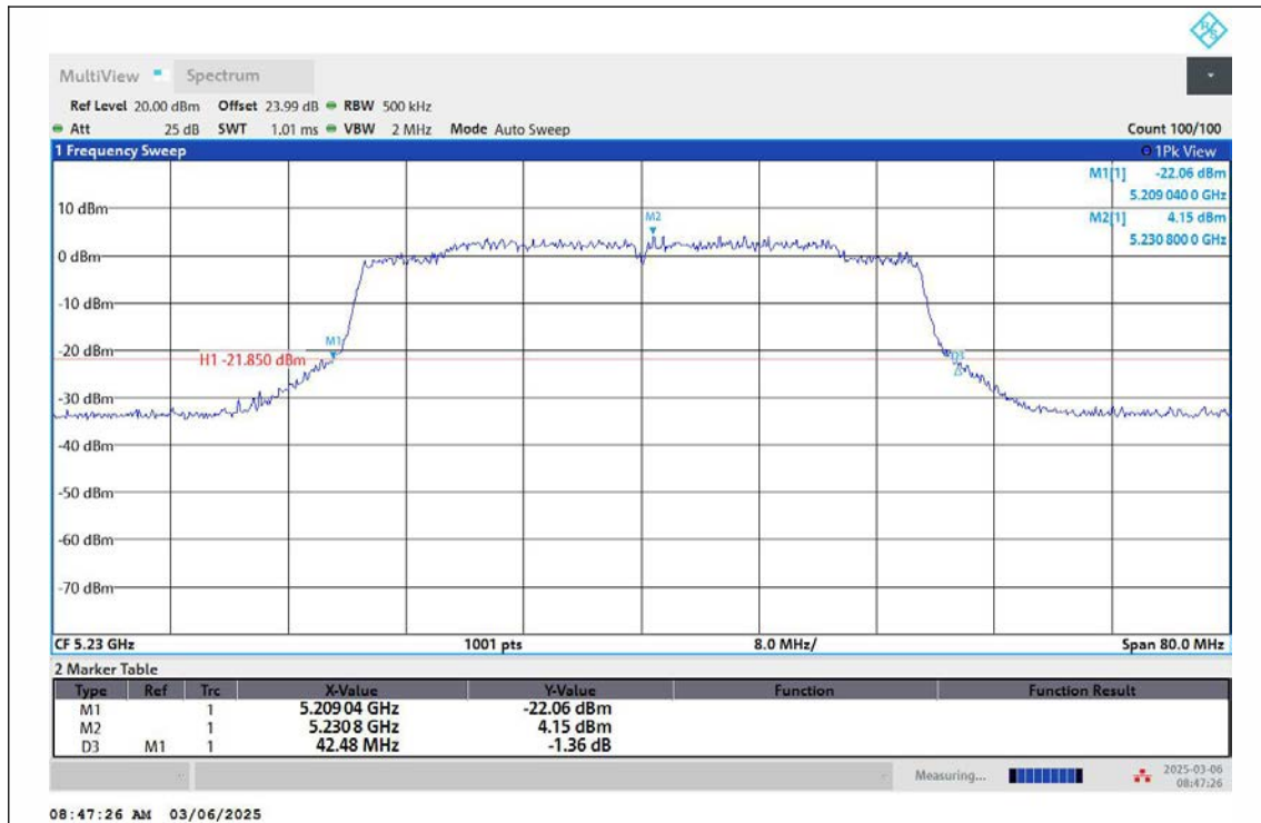
11AX40MIMO-Ant2-5230
