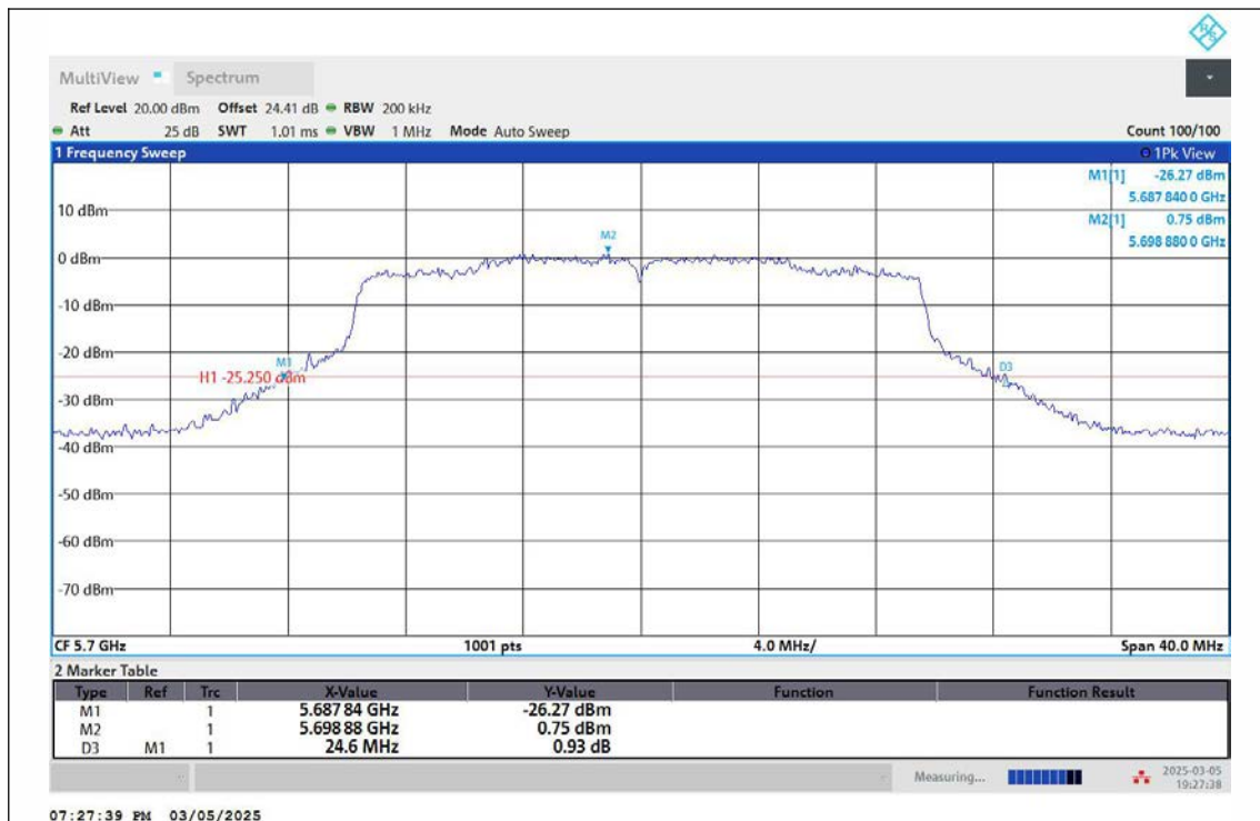
11AX20MIMO-Ant2-5700
