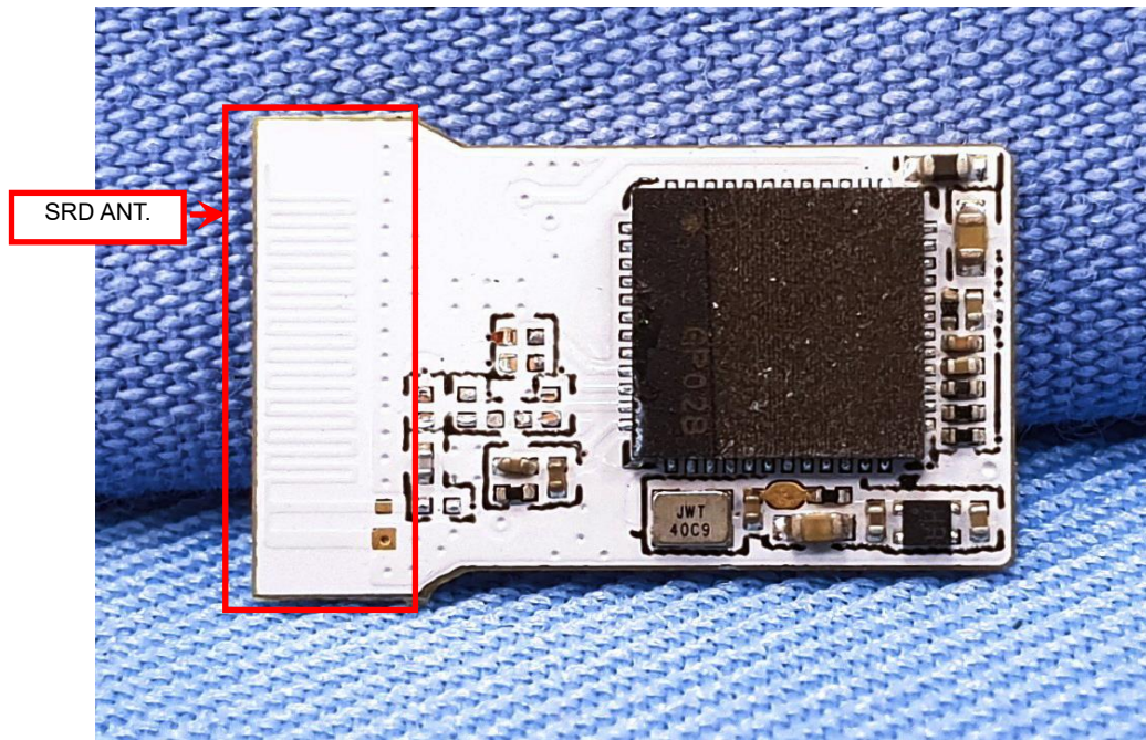
EUT Photo (5)
