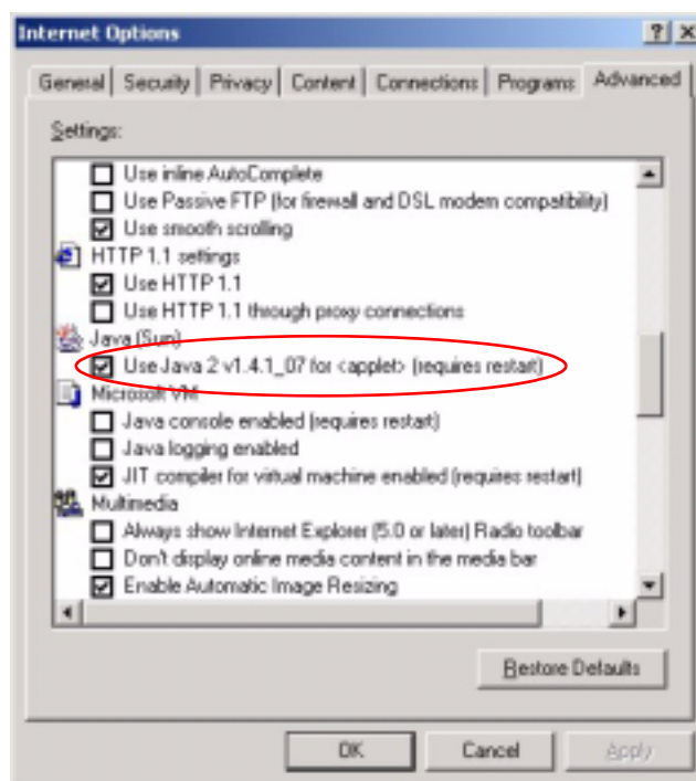
Figure 78 Java (Sun)
