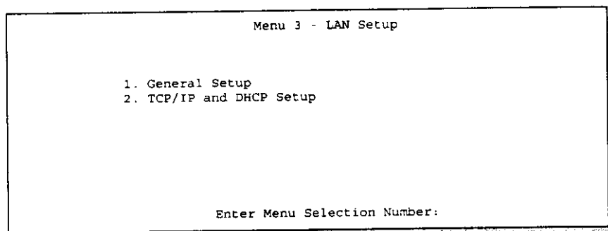
Figure2-9 Menu 3 - LAN Setup
