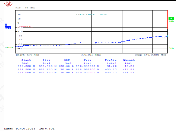
FDD12HighRange_10MHz_QPSK_OneRB low
