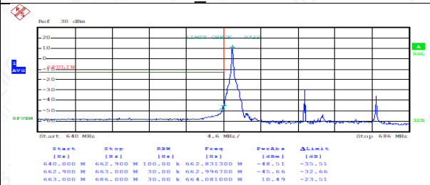
FDD71LowRange_20MHz_QPSK_OneRB_low
