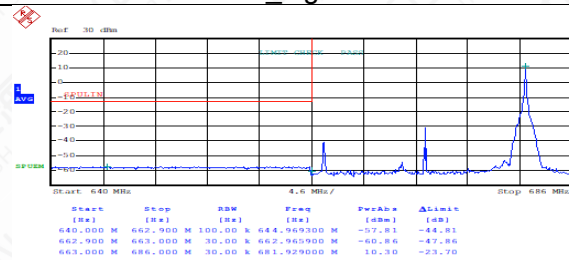
FDD71LowRange_20MHz_QPSK_OneRB_high
