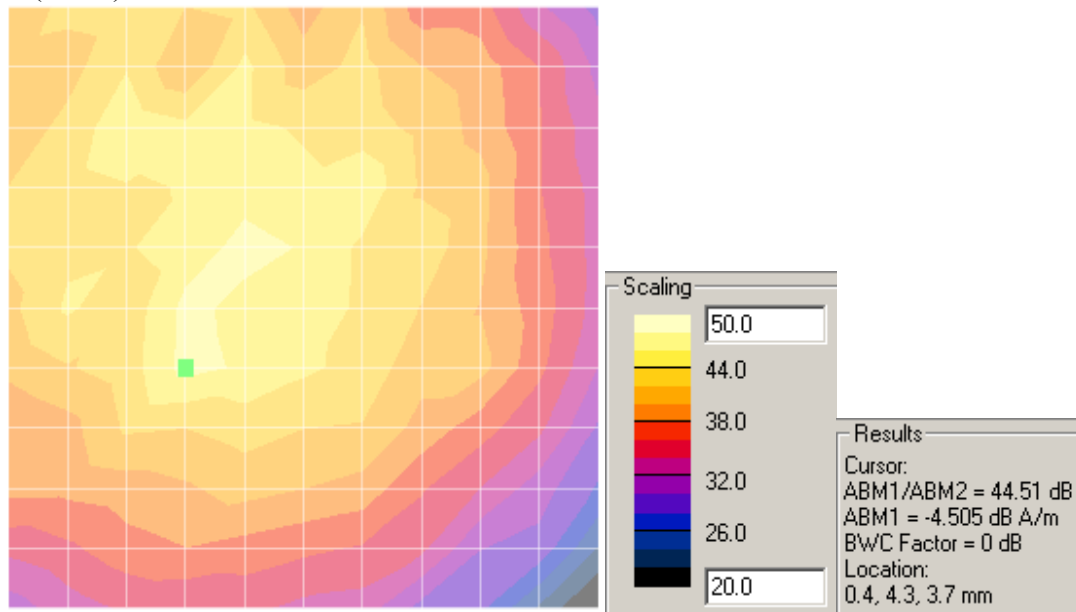
Z (Axial) – SNR
