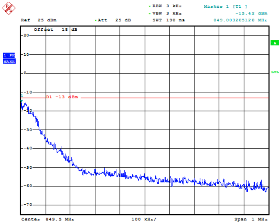
(Plot B5: GSM 850MHz Channel = 251)
