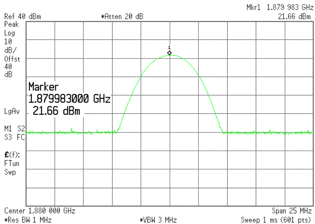
(Plot E6.2:EGPRS 1900MHz Channel = 661)
