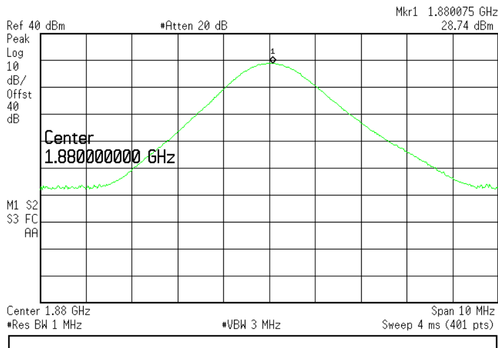
(Plot E6:GSM 1900MHz Channel = 661)
