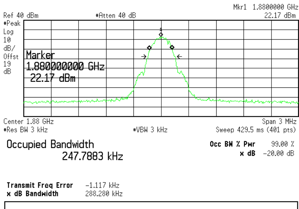
(Plot E3.1: GPRS 1900MHz Channel = 661)
