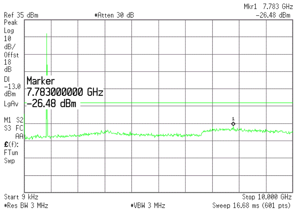
(Plot N4.:EGPRS 850MHz Channel = 190, 9KHz to 10GHz)
