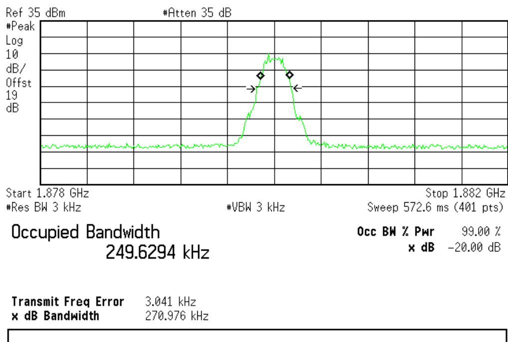
(Plot E3.2: EGPRS 1900MHz Channel = 661)
