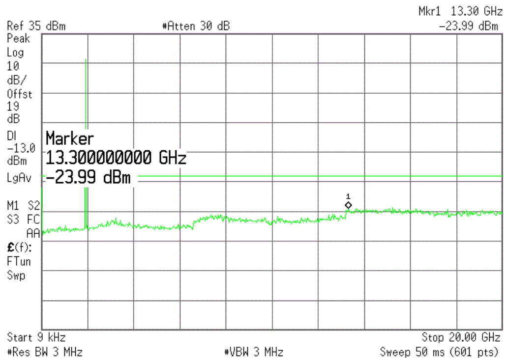
(Plot P4.:EGPRS 1900MHz Channel = 512, 9KHz to 20GHz)
