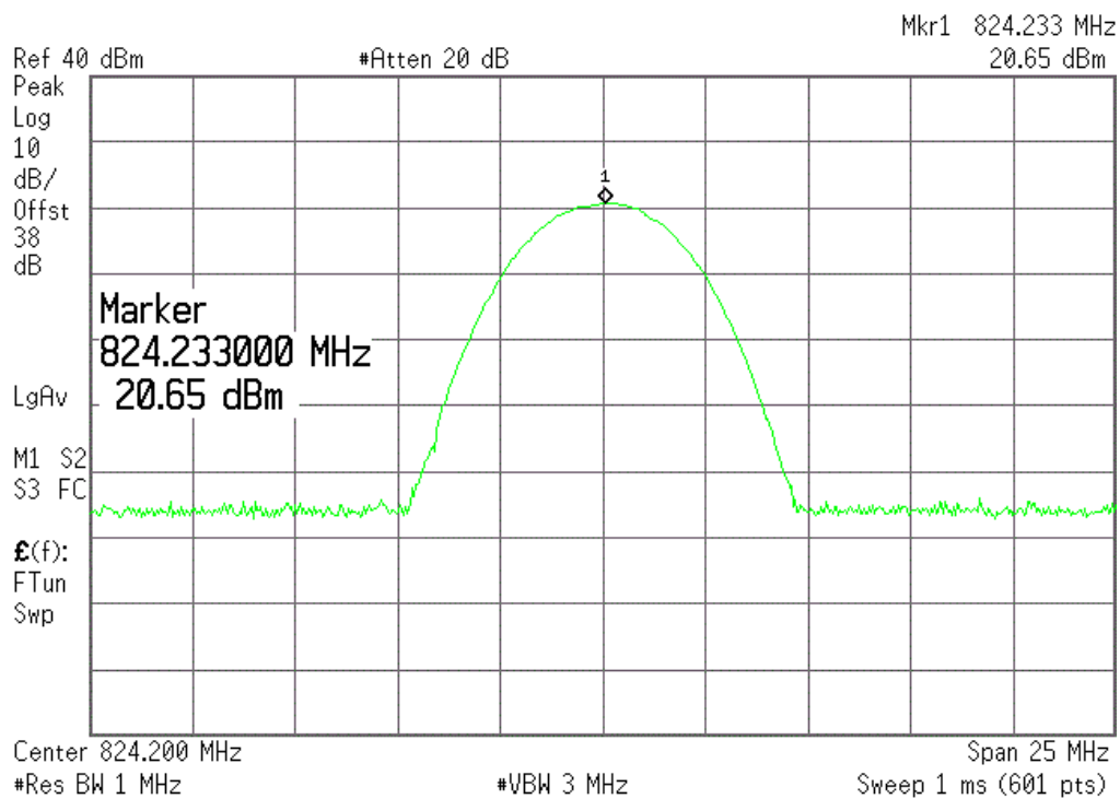
(Plot A6.2:EGPRS 850MHz Channel = 128)
