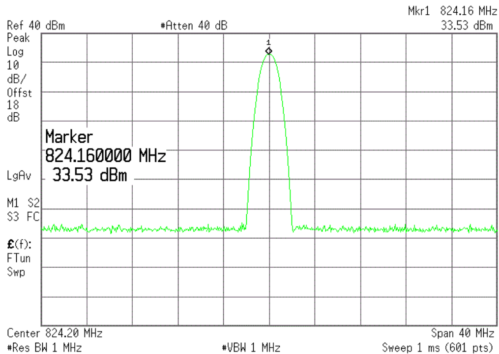
(Plot E1: GPRS 850MHz Channel = 128)
