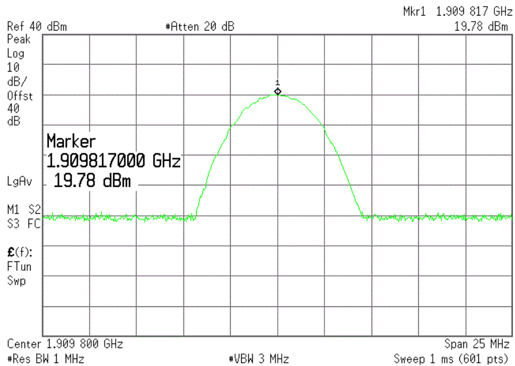
(Plot F6.2:EGPRS 1900MHz Channel = 810)
