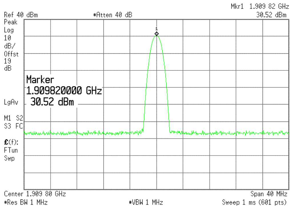
(Plot F2: GSM 1900MHz Channel = 810)
