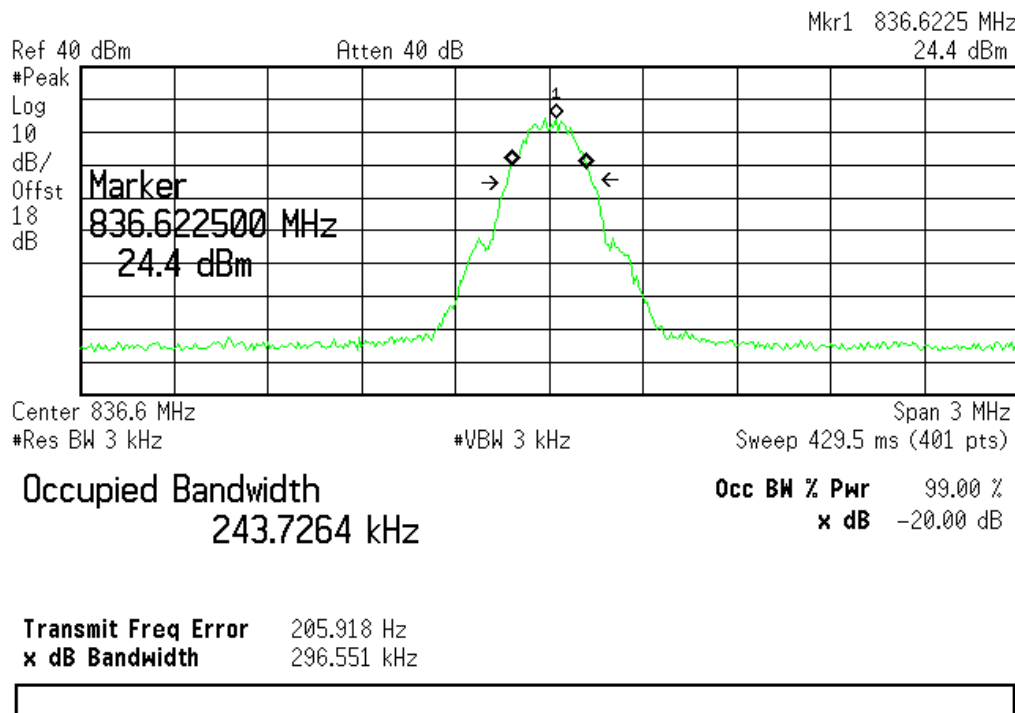
(Plot B3: GSM 850MHz Channel = 190)
