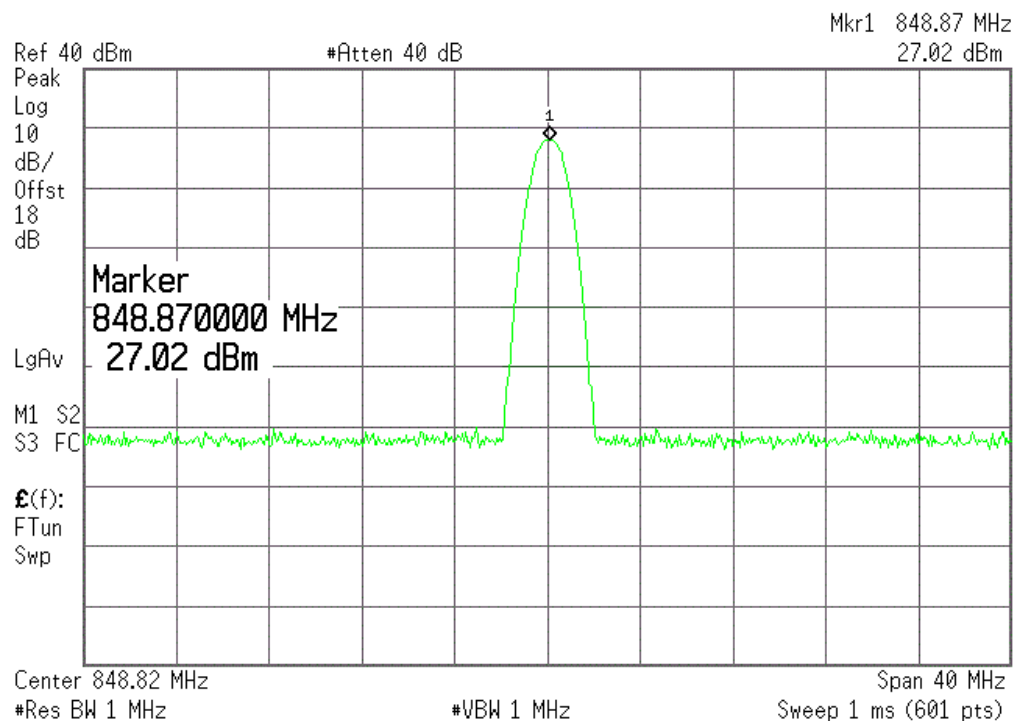
(Plot O2:EGPRS 850MHz Channel = 251)
