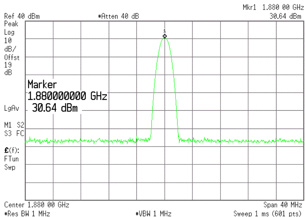
(Plot E2: GSM 1900MHz Channel = 661)
