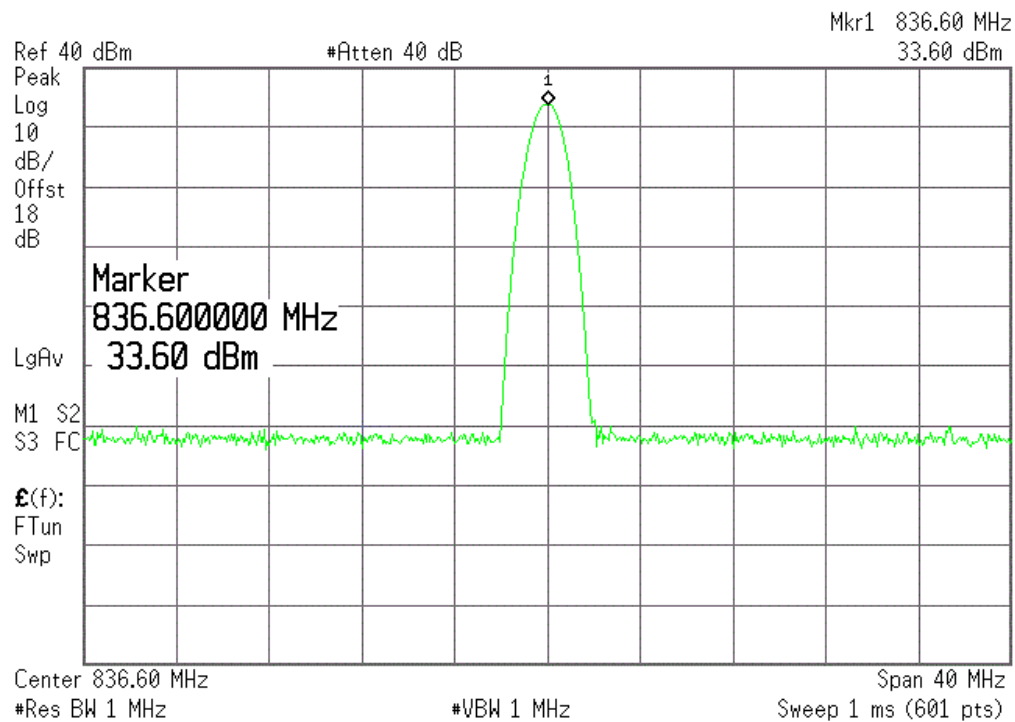
(Plot B2: GSM 850MHz Channel = 190)
