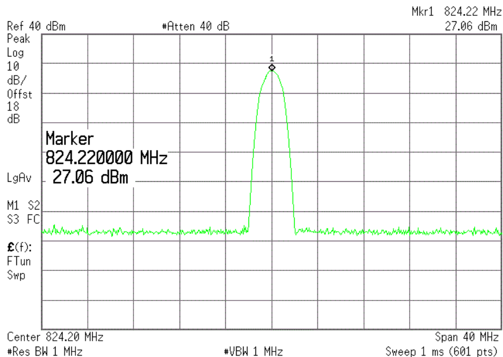
(Plot M2:EGPRS 850MHz Channel = 128)
