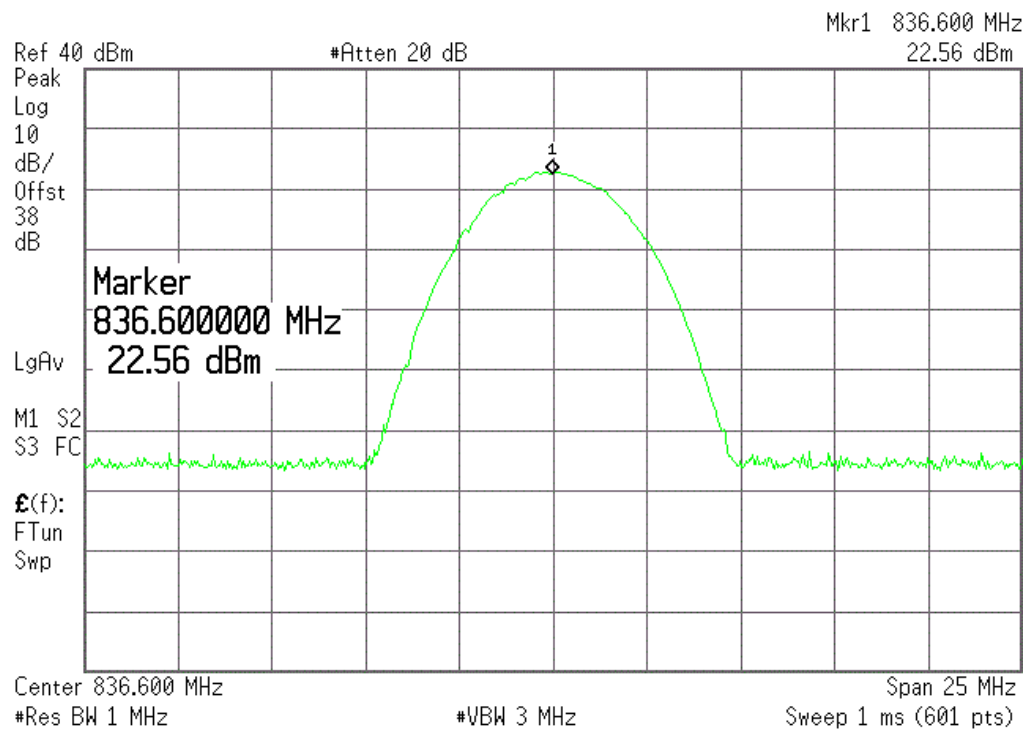
(Plot B6.2:EGPRS 850MHz Channel = 190)
