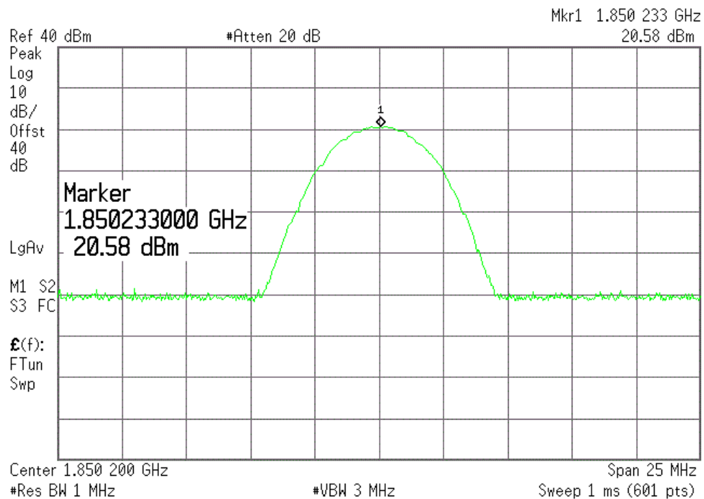
(Plot D6.2:EGPRS 1900MHz Channel = 512)
