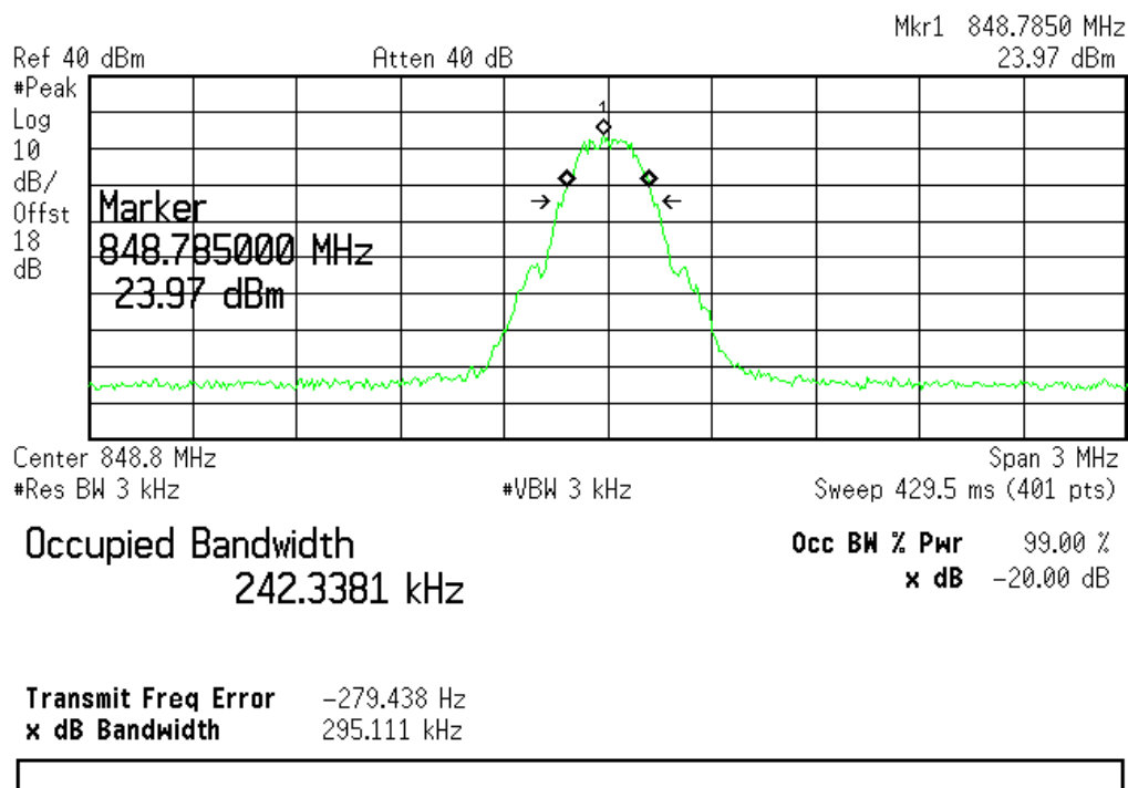
(Plot C3: GSM 850MHz Channel = 251)
