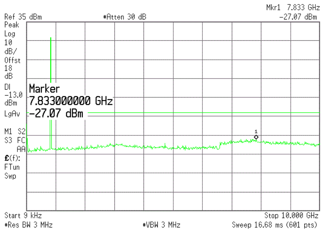
(Plot O4.:EGPRS 850MHz Channel = 251, 9KHz to 10GHz)
