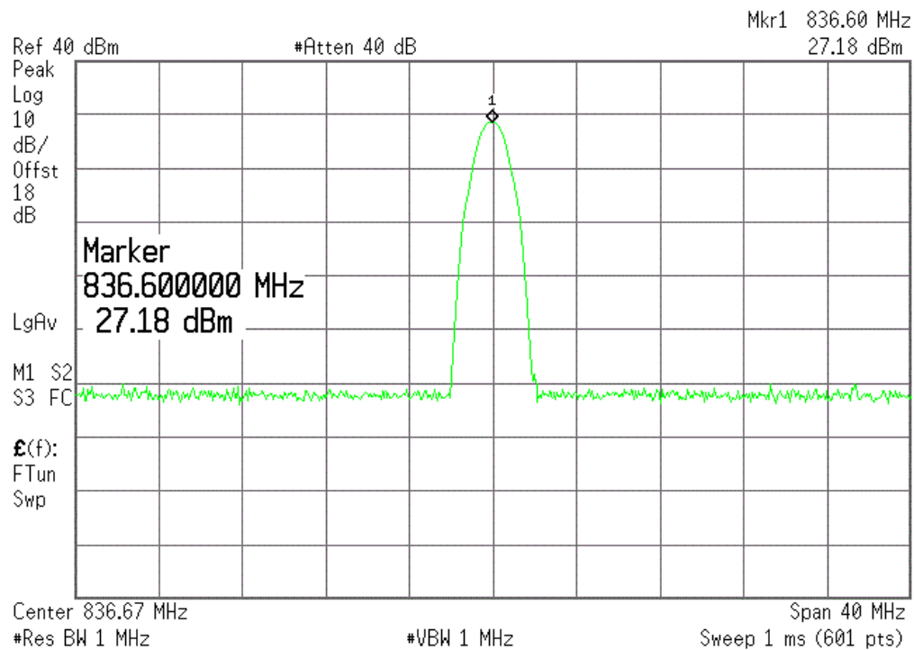
(Plot N2:EGPRS 850MHz Channel = 190)
