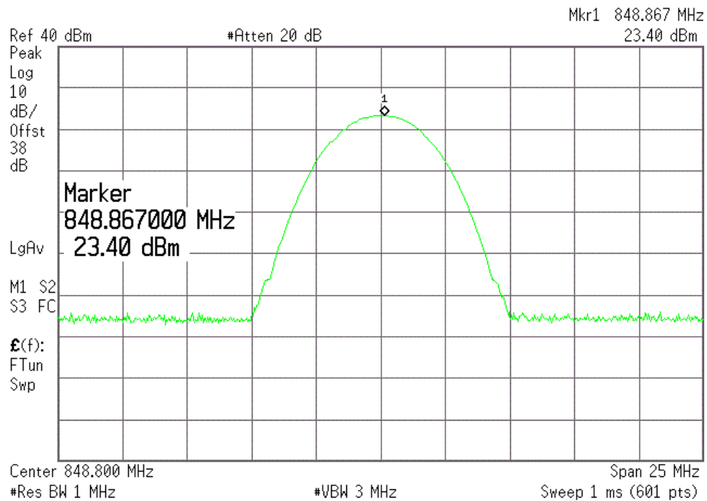
(Plot C6.2:EGPRS 850MHz Channel = 251)
