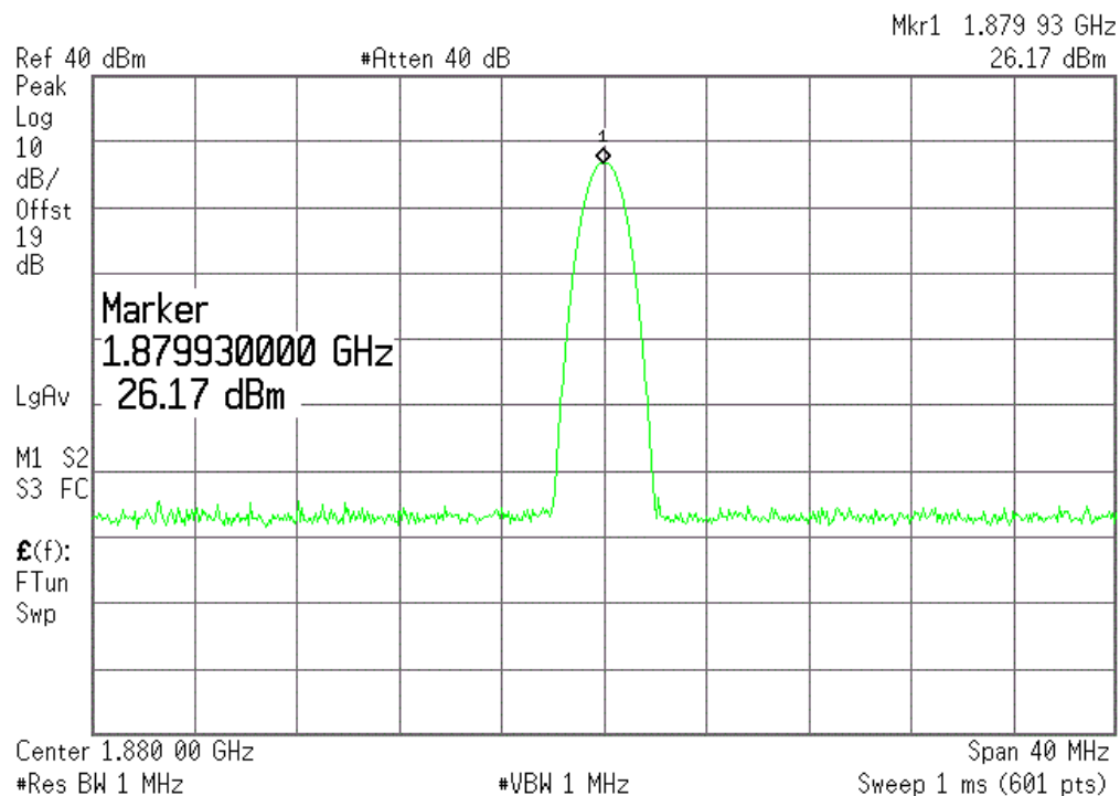
(Plot Q2:EGPRS 1900MHz Channel = 661)
