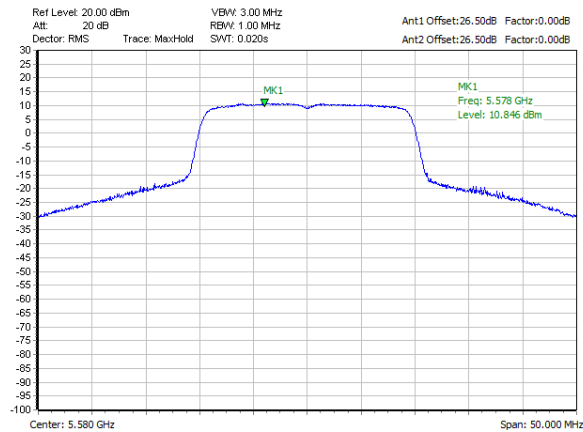
MIMO Ant. 4+5
