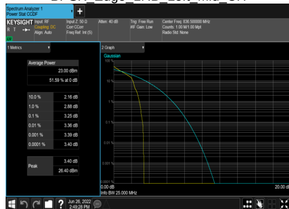
B7_N5(20M)_DFT-s-OFDM_PI_2-BPSK Edge 1RB Left Mid CH
