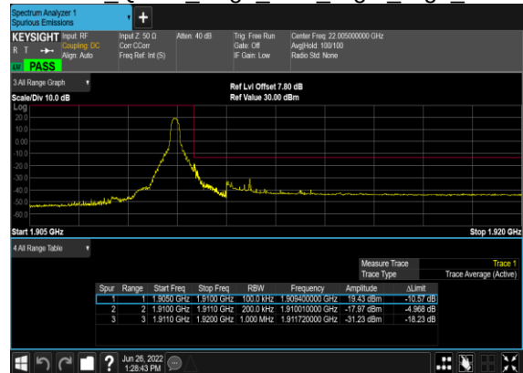
B7_N2(20M)_DFT-s- OFDM QPSK Edge 1RB Right High CH
