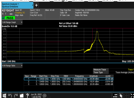
B7_N2(20M)_DFT-s-OFDM BPSK Edge 1RB Left Low CH
