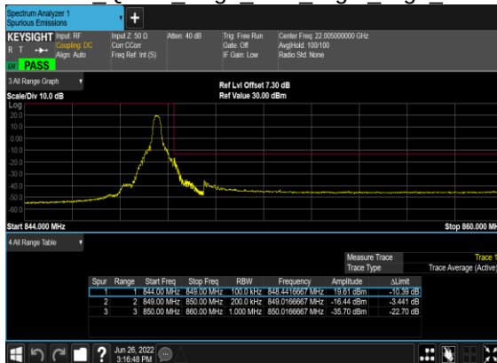
B7_N5(20M)_DFT-s- OFDM QPSK Edge 1RB Right High CH
