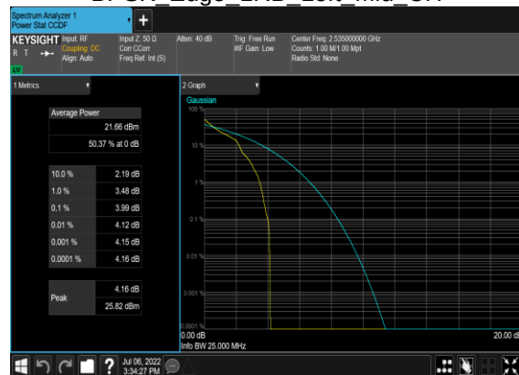
N7(20M)_DFT-s-OFDM_PI_2-BPSK Edge 1RB Left Mid CH
