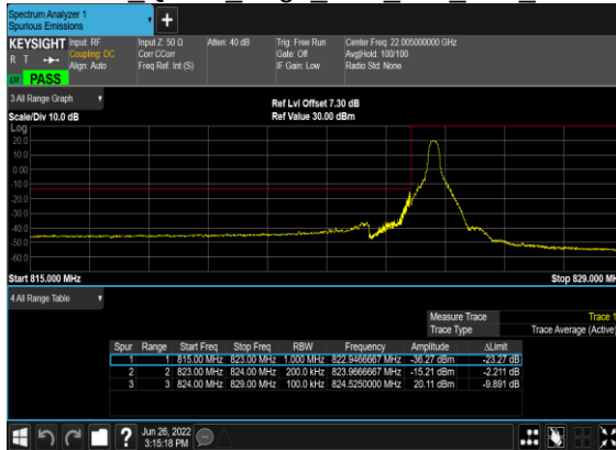
B7_N5(20M)_DFT-s- OFDM QPSK Edge 1RB Left Low CH
