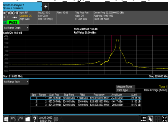
B7_N5(20M)_DFT-s-OFDM BPSK Edge 1RB Left Low CH
