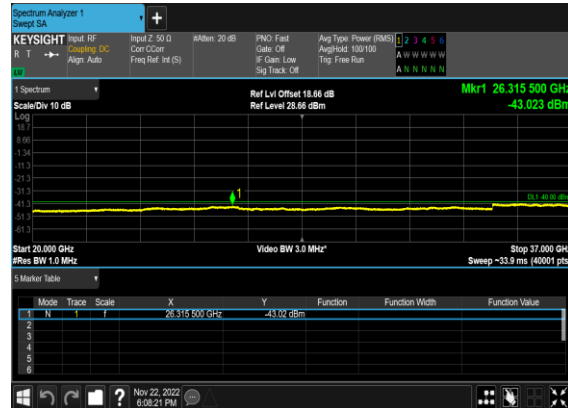
N48(40M)_CP- OFDM_QPSK_Edge_1RB_Left_Low_CH
