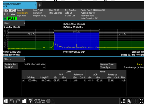
N48(100M)_DFT-s-OFDM_PI_2- BPSK Edge 1RB Left High CH
