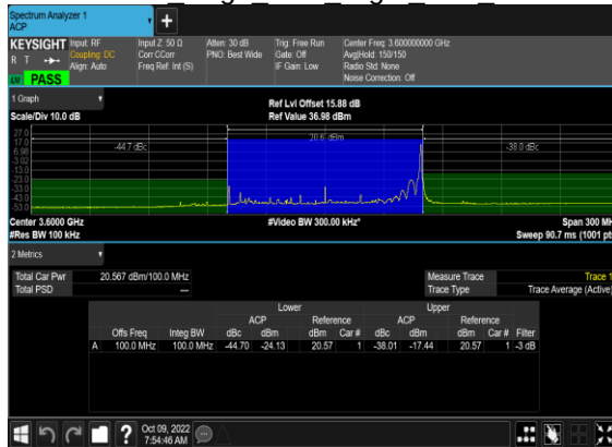
N48(100M)_DFT-s-OFDM_PI_2-BPSK Edge 1RB Right Low CH
