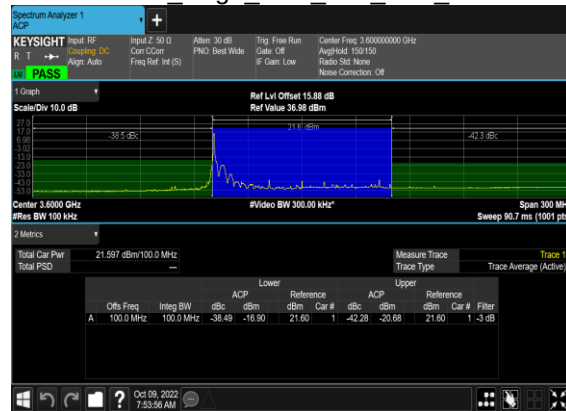
N48(100M)_DFT-s-OFDM_PI_2-BPSK Edge 1RB Left Low CH
