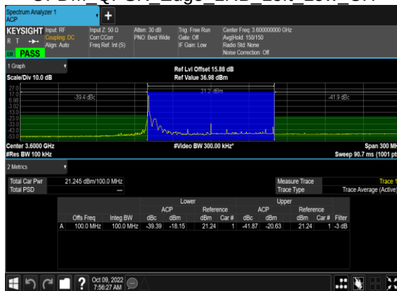
N48(100M)_DFT-s-OFDM QPSK Edge 1RB Left Low CH
