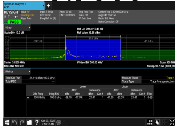
N48(100M)_DFT-s-OFDM_PI_2- BPSK Edge 1RB Left Mid CH
