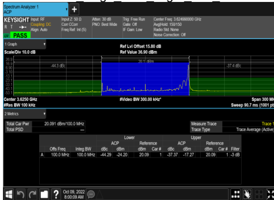
N48(100M)_DFT-s-OFDM_PI_2- BPSK Edge 1RB Right Mid CH
