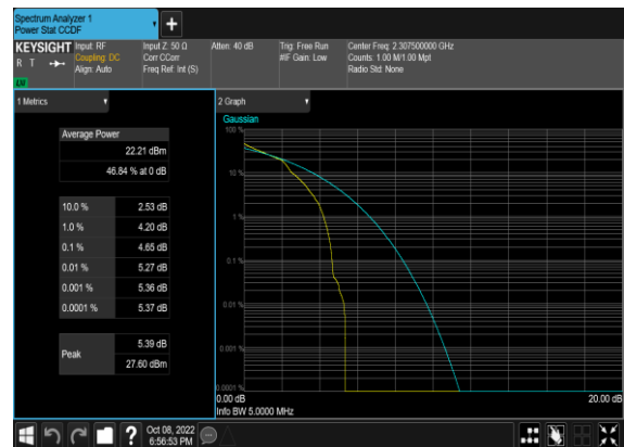
N30(5M)_DFT-s-OFDM_QPSK_Edge_1RB_Left_Low_ CH
