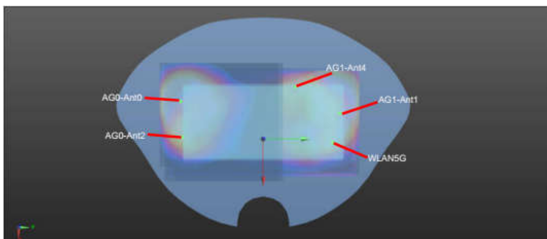
Extremity_Front 0mm
