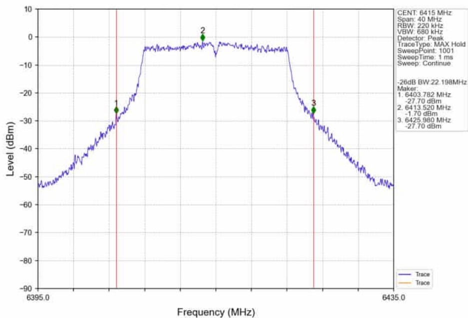
802.11a_HCH_6415MHz_Ant4_NTNV
