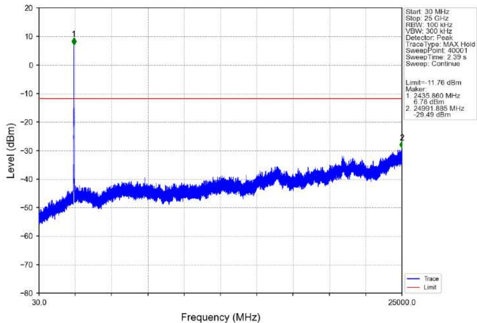
802.11ax(HEW20)_MCH_2437MHz_SU_/_Ant3 (MIMO)_NTNV
