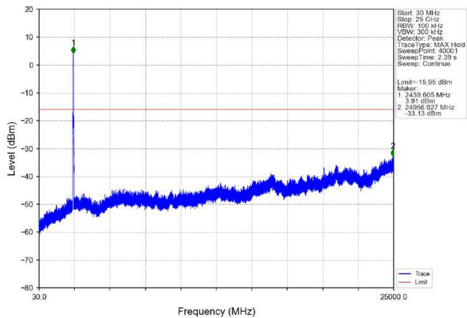
802.11ax(HEW40)_MCH_2437MHz_SU_/_Ant3 (MIMO)_NTNV
