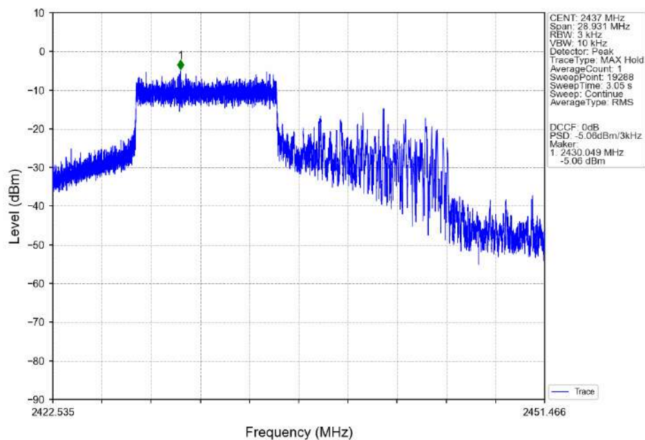
802.11ax(HEW20)_MCH_2437MHz_RU106_Left_Ant3 (MIMO)_NTNV
