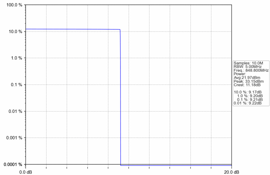
GSM850_GSM_HCH_848.8MHz_GSM_NTNV
