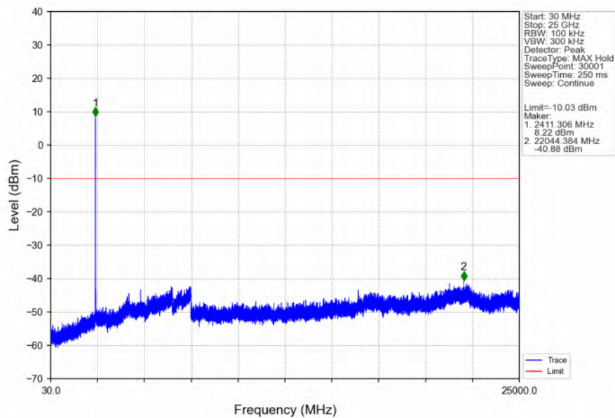
802.11b_LCH_2412MHz_Ant6 (SISO)_NTNV
