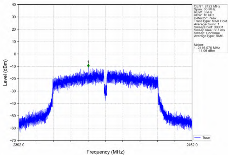
802.11n(HT40) LCH 2422MHz Ant6 (SISO) NTN
