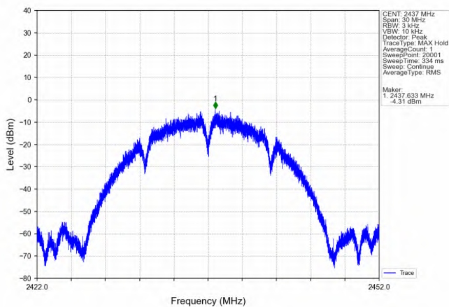
802.11b MCH 2437MHz Ant6 (SISO) NTN
