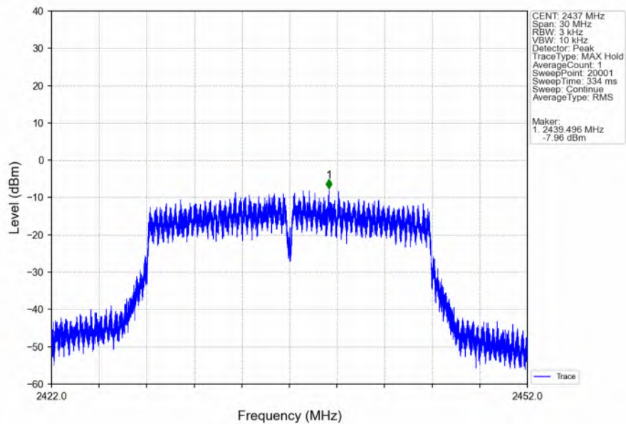
802.11n(HT20) MCH_2437MHz_Ant6 (SISO)_NTNV
