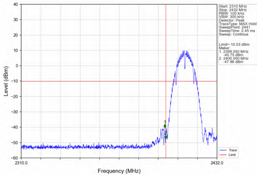
802.11b_LCH_2412MHz_Ant6 (SISO)_NTNV
