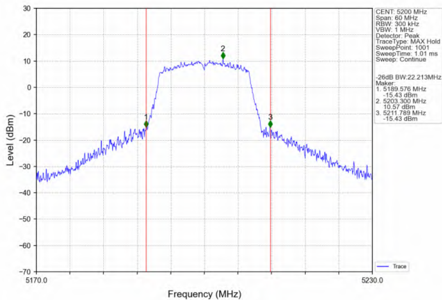
802.11a_MCH_5200MHz_Ant6_NTNV
