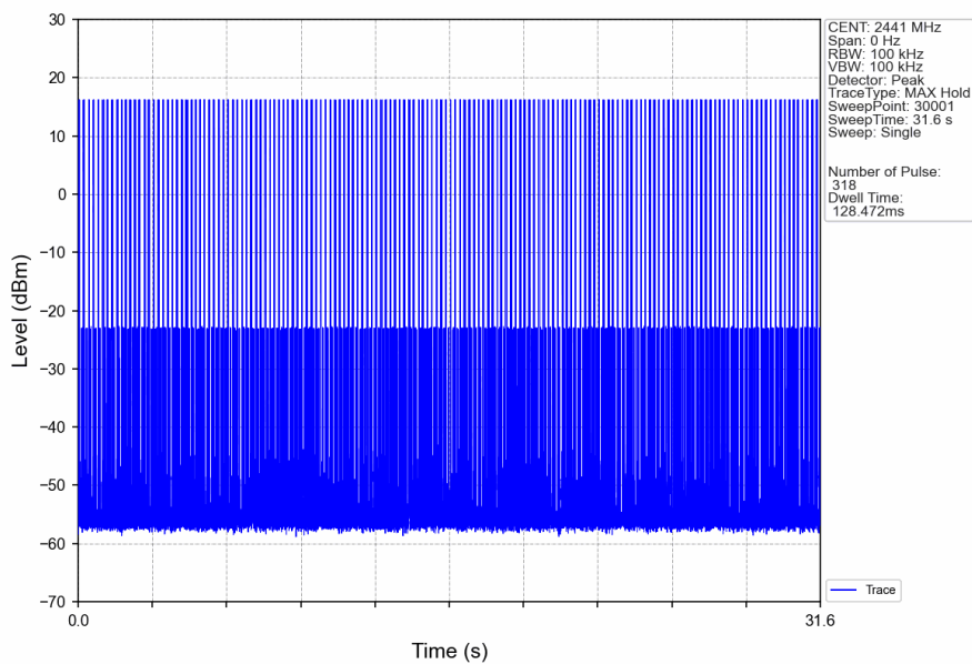
Pi/4DQPSK_2DH1_HOPP_Ant6_NTNV
