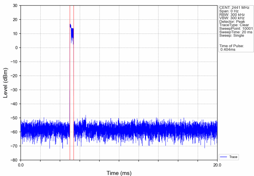
Pi/4DQPSK_2DH1_HOPP_Ant6_NTNV
