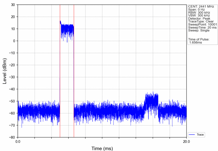
Pi/4DQPSK_2DH3_HOPP_Ant6_NTNV
