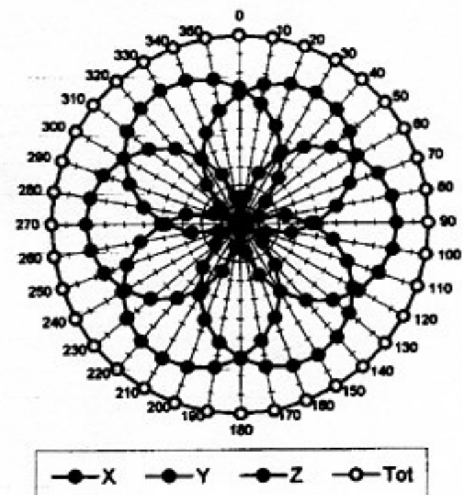
f = 900 MHz, TEM cell if110
