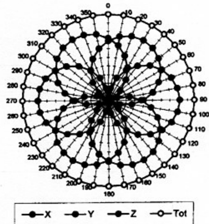
f = 100 MHz, TEM cell if110
