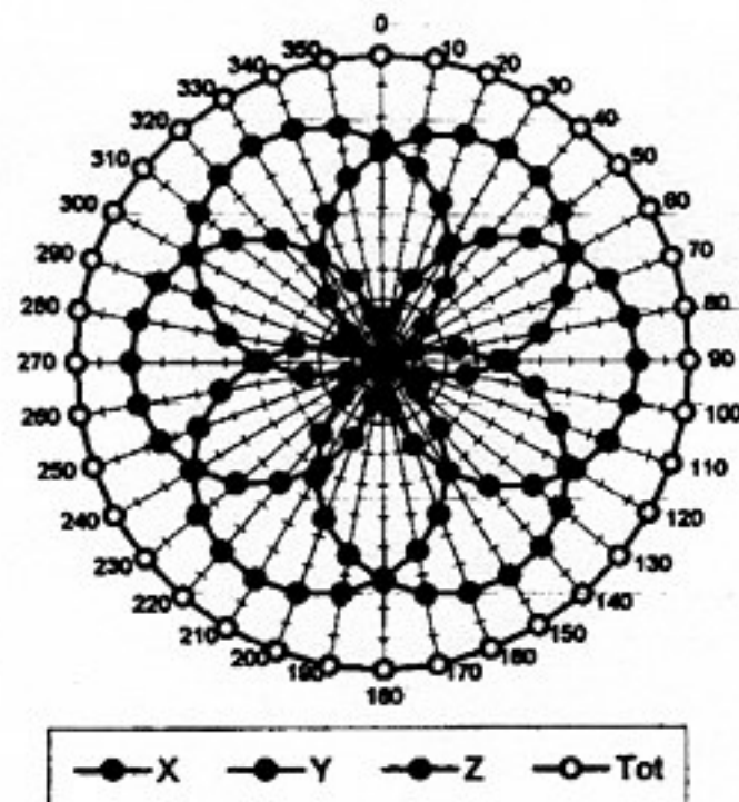
f = 300 MHz, TEM cell if110
