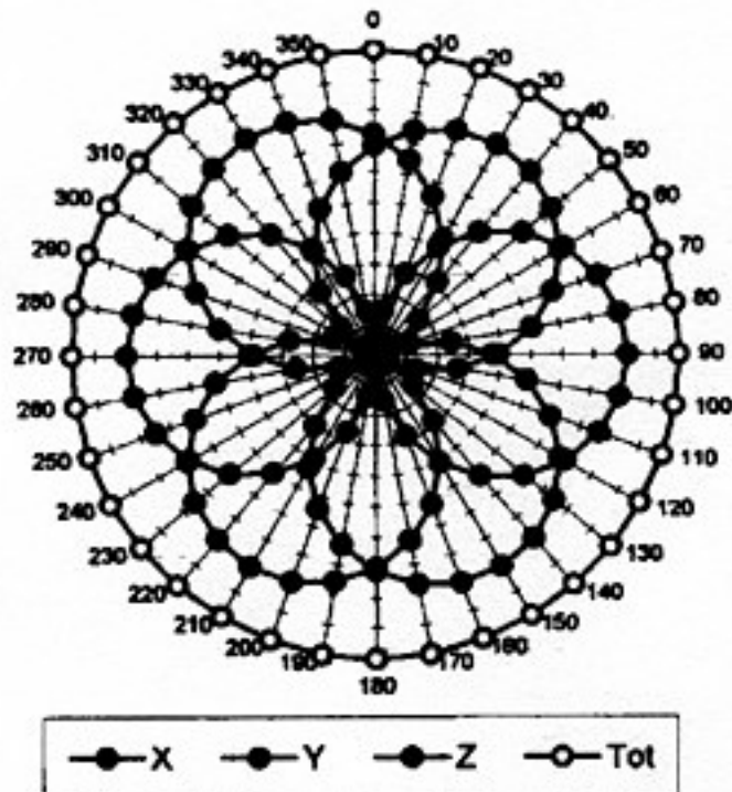
f = 30 MHz, TEM cell if110
