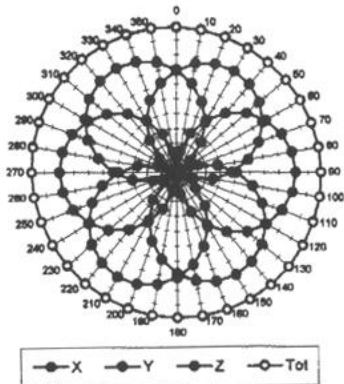
f = 300 \text{ MHz} , TEM cell I#110
