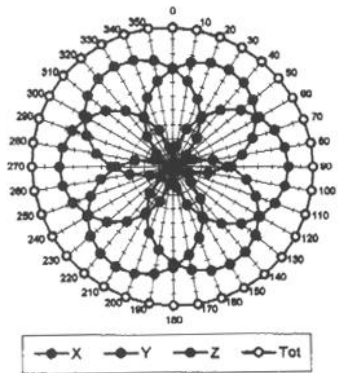
f = 900 \text{ MHz} , TEM cell I#110
