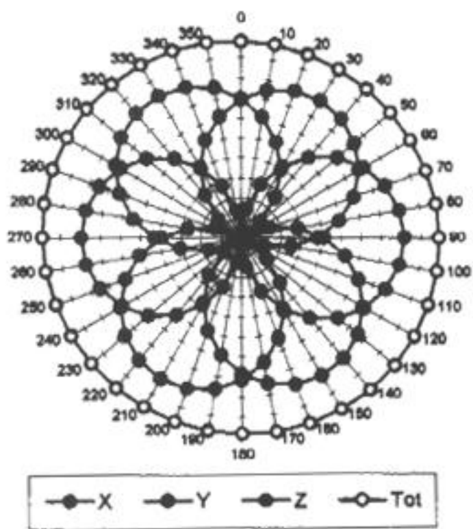
f = 900 \text{ MHz} , TEM cell I#110
