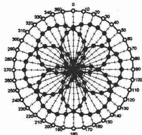
f = 100 \text{ MHz} , TEM cell if110
