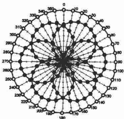
f = 300 \text{ MHz} , TEM cell if110
