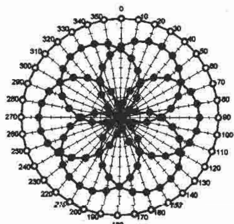
f = 900 \text{ MHz} , TEM cell if110
