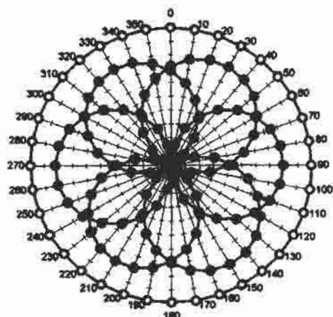
f = 30 \text{ MHz} , TEM cell if110
