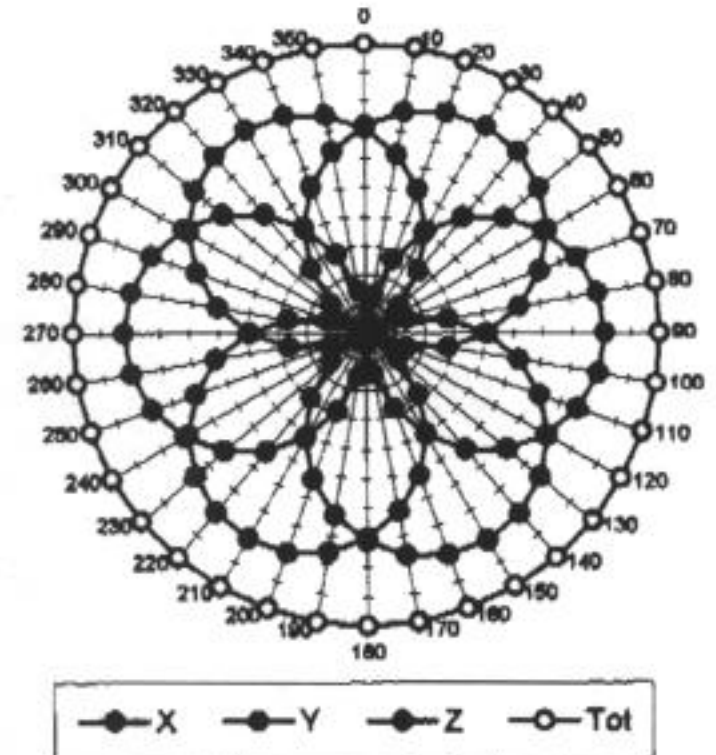
f = 900 MHz, TEM cell if110
