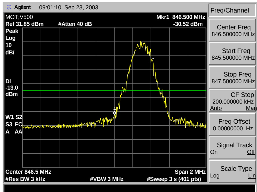
GSM 850 B* Min. Block Edge
