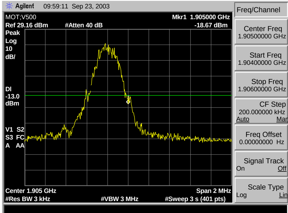
GSM 1900 C4 Max Block Edge
