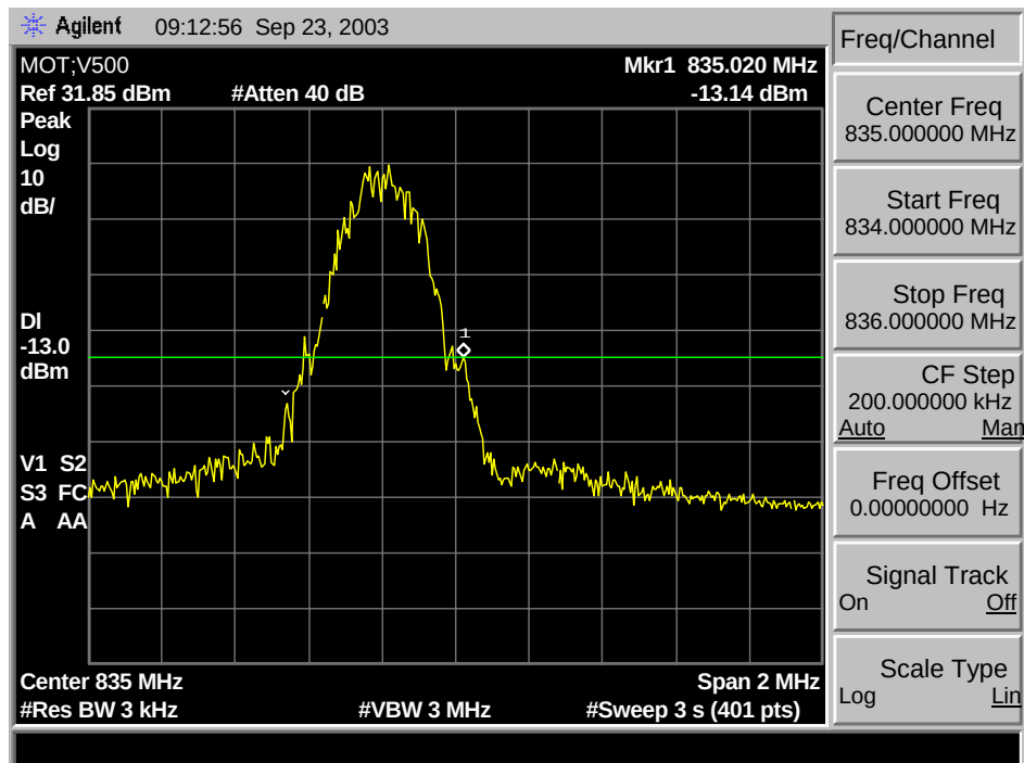
GSM 850 A Max Block Edge
