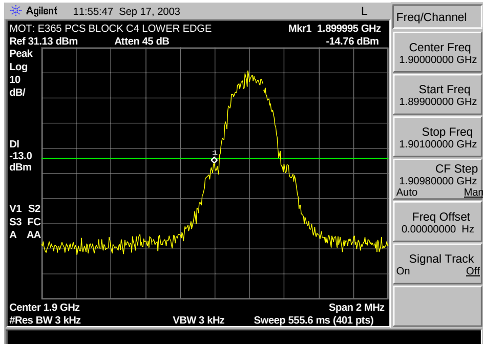
GSM 1900 C4 Min. Block Edge
