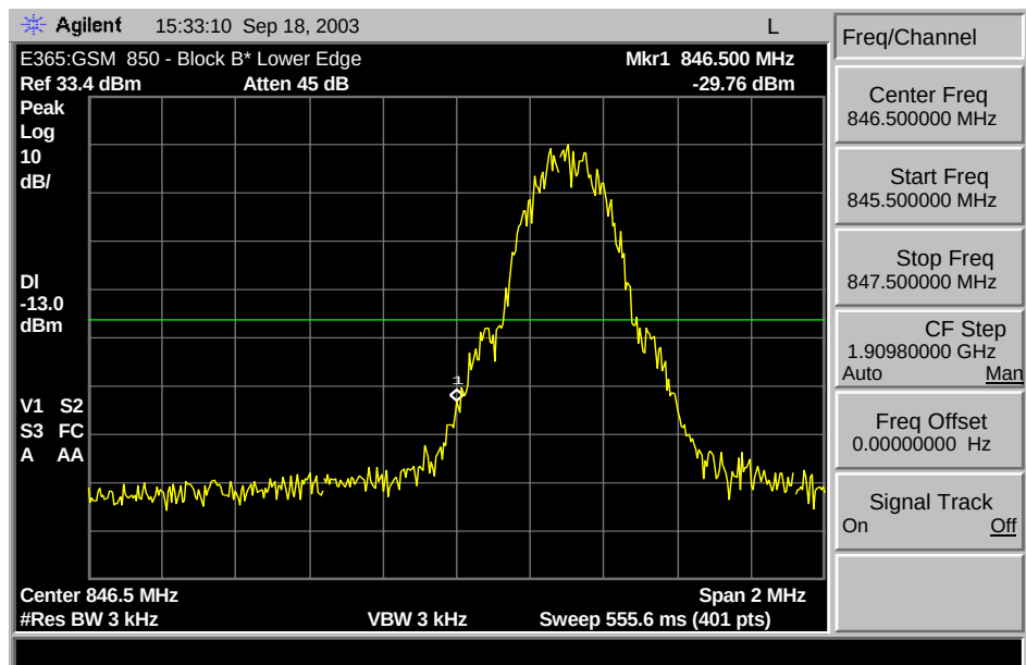
GSM 850 B* Min. Block Edge
