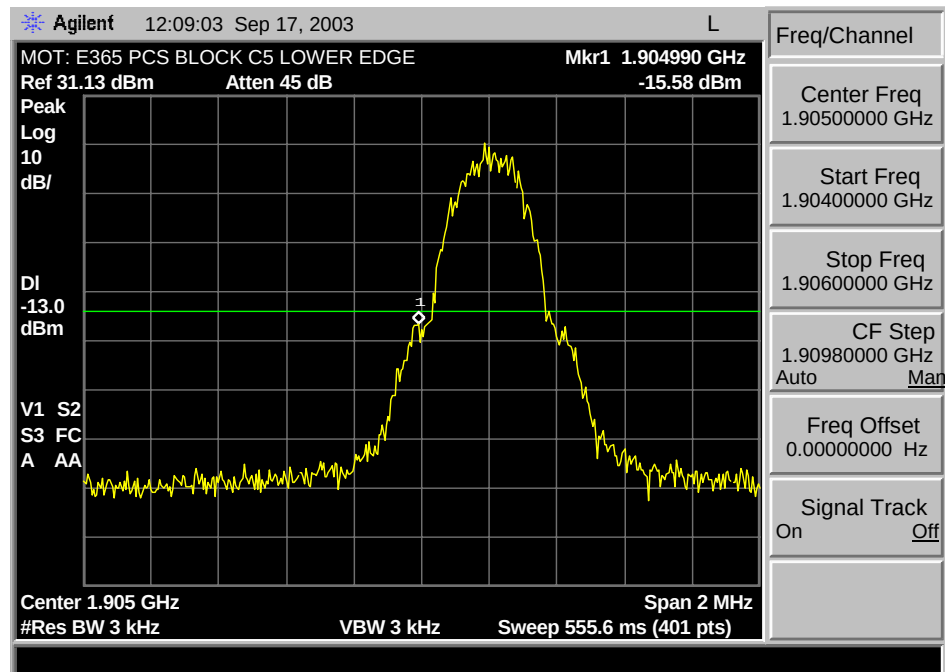
GSM 1900 C5 Min. Block Edge
