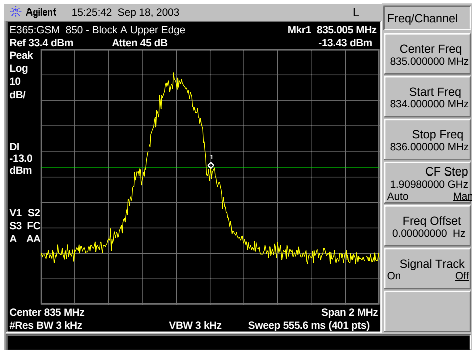
GSM 850 A Max Block Edge
