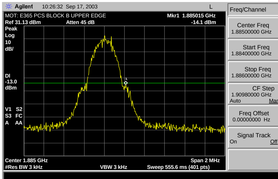
GSM 1900 B Max Block Edge
