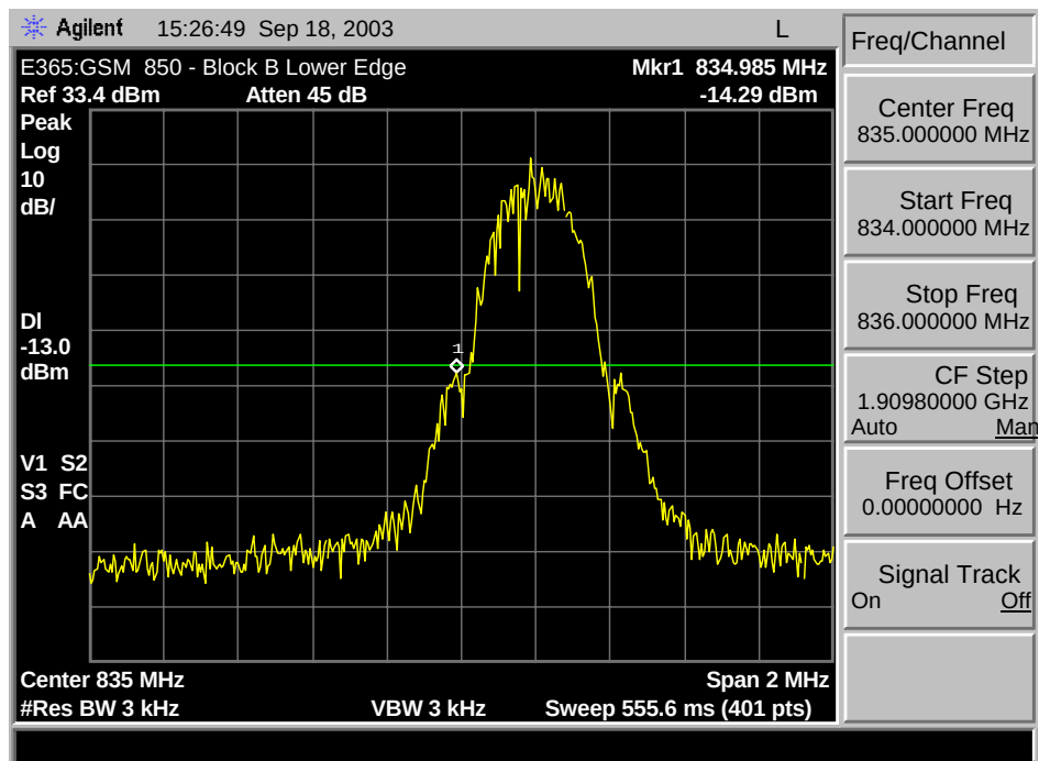
GSM 850 B Min. Block Edge
