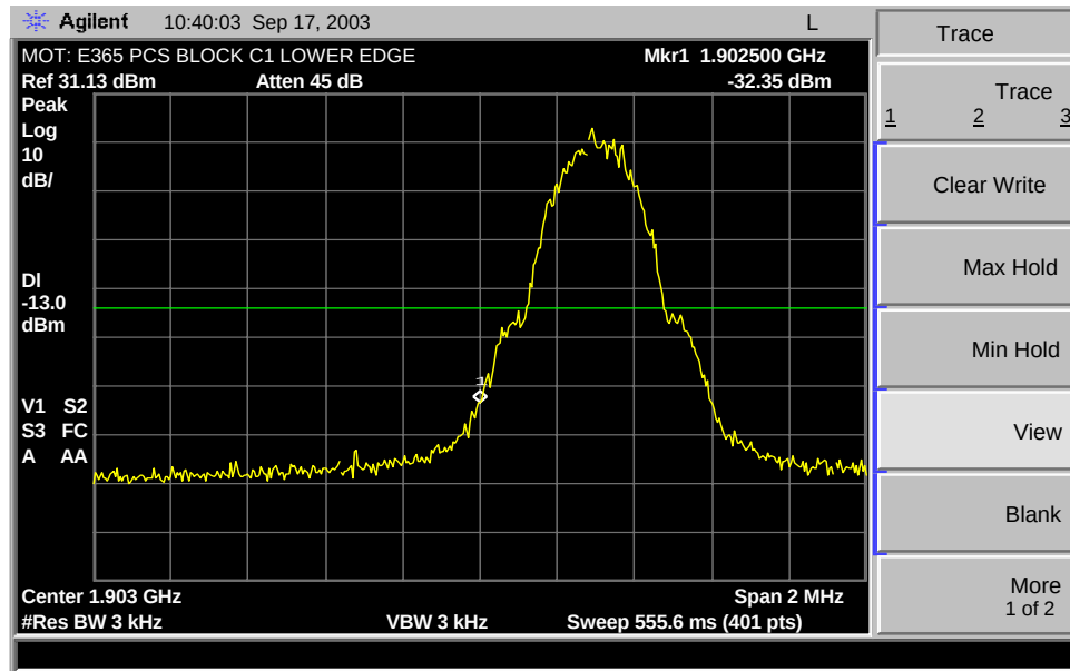
GSM 1900 C1 Min. Block Edge
