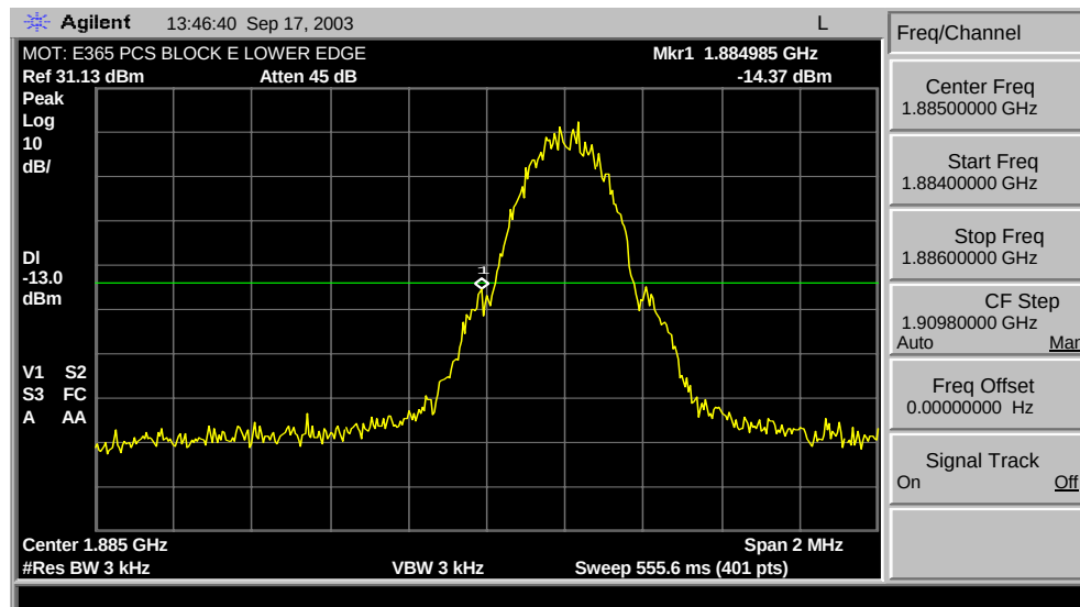
GSM 1900 E Min. Block Edge
