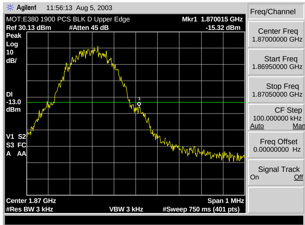
GSM 1900 D Max Block Edge
