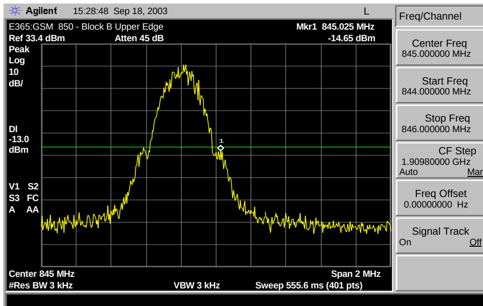
GSM 850 B Max Block Edge
