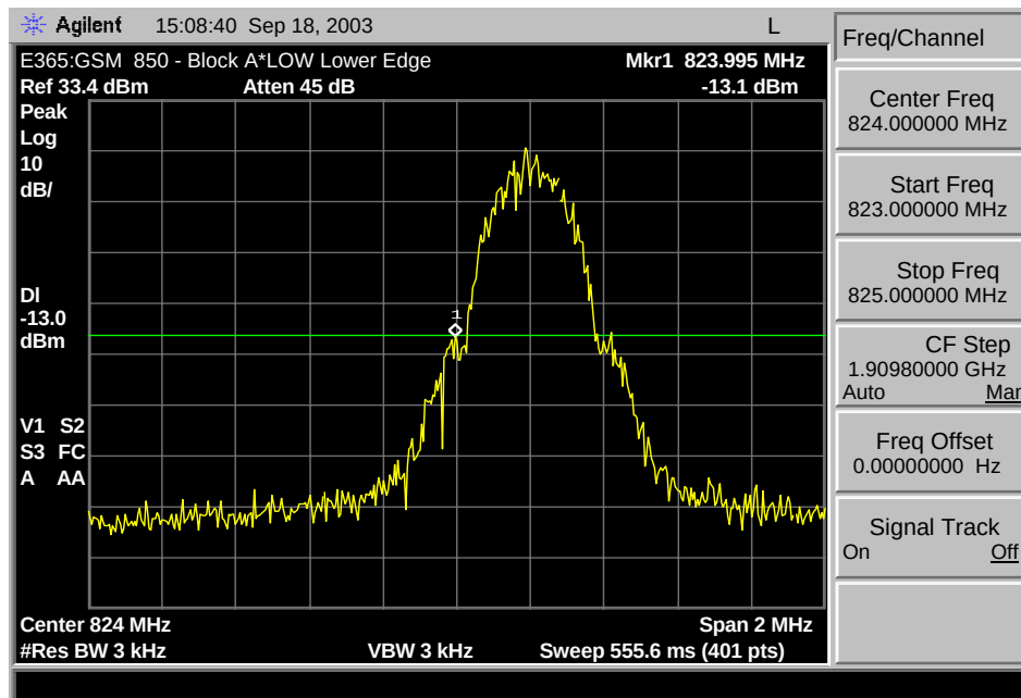
GSM 850 A*(Lower) Min. Block Edge
