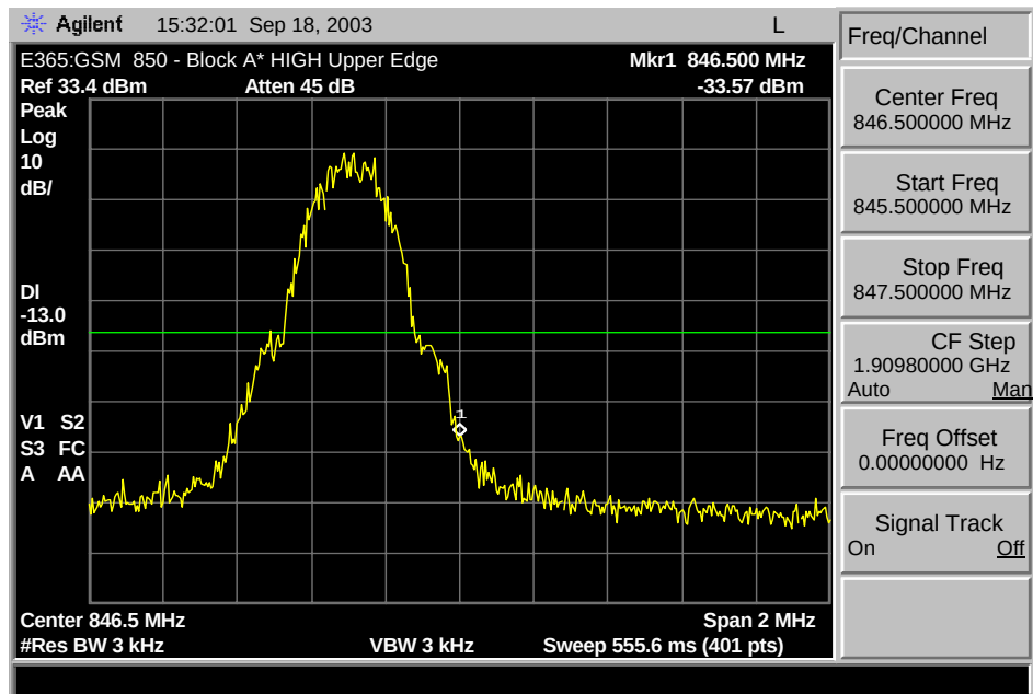
GSM 850 A*(Upper) Max Block Edge
