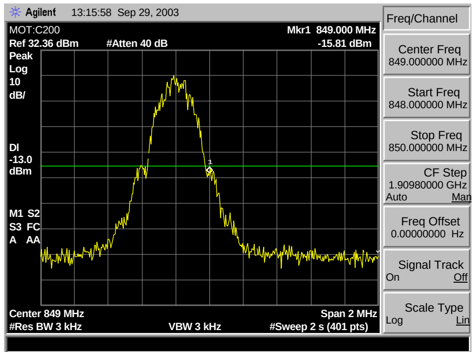
GSM 850 Max Band Edge
