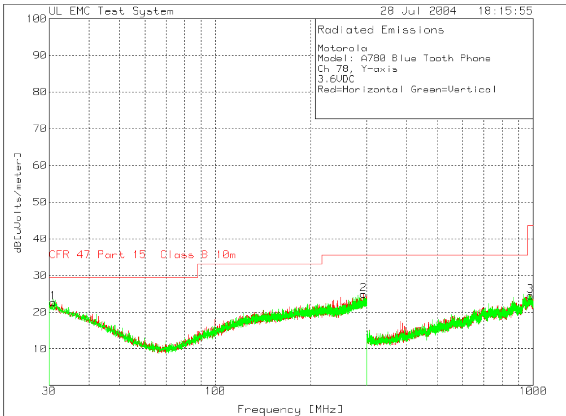
30MHz – 1000MHz Ch78 Y-Axis
