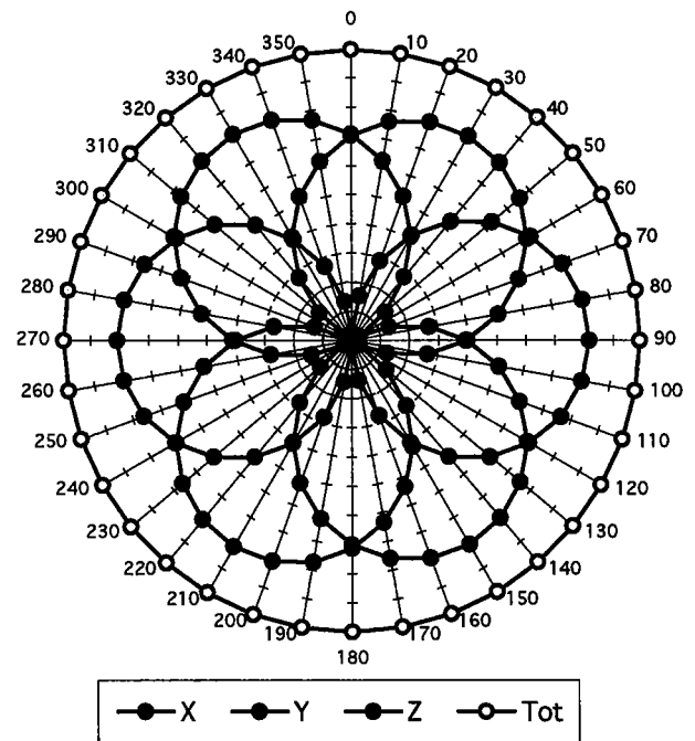
f = 100 \text{ MHz} , TEM cell ifi110
