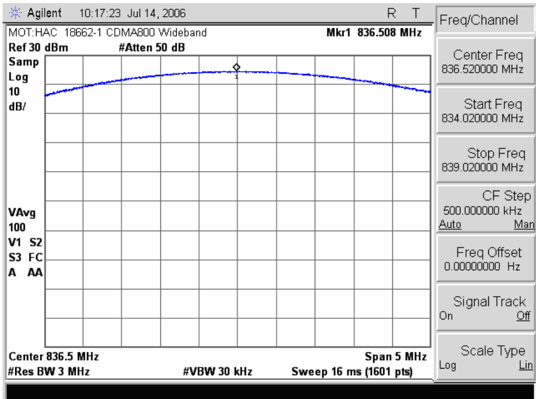
CDMA800 CH 384 (836.52) WIDEBAND
