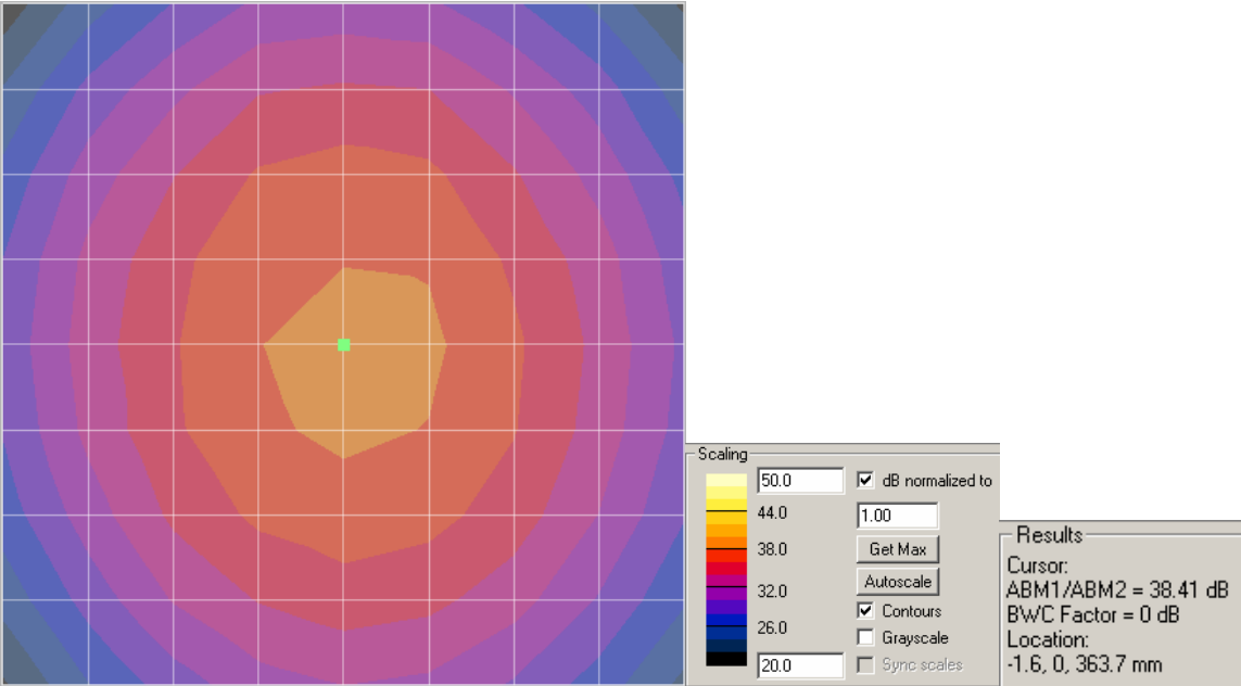
Axial - SNR
