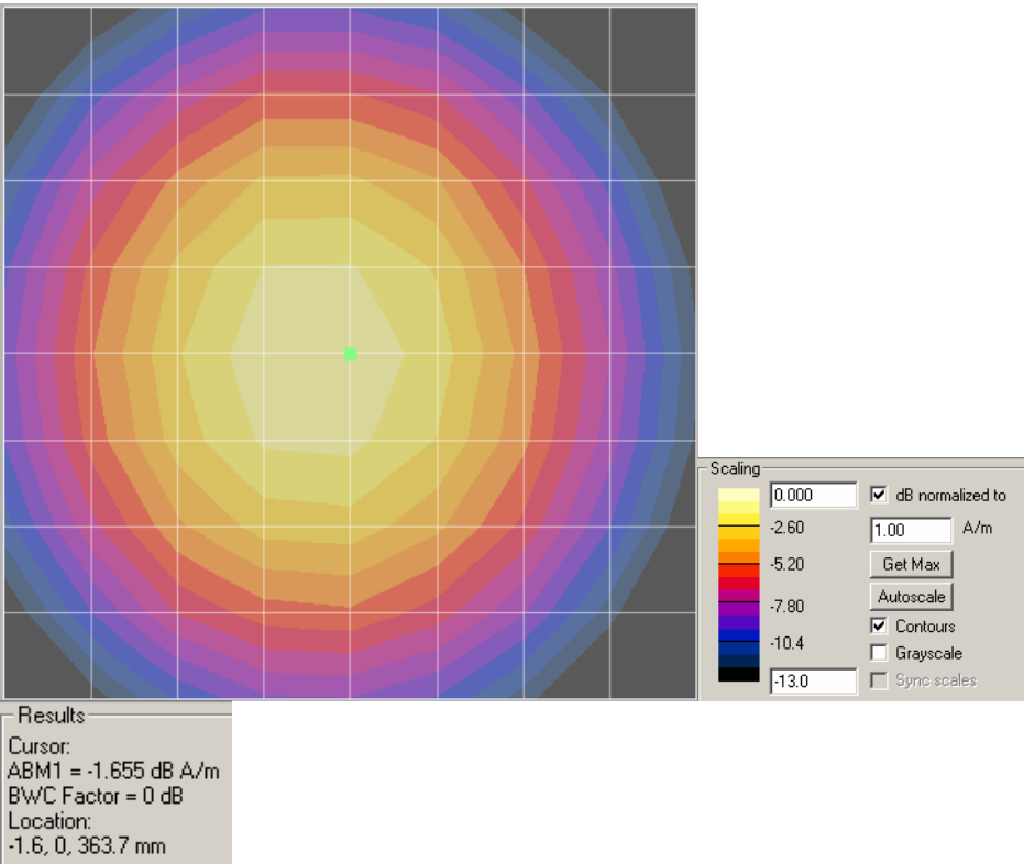
Axial - ABM1
