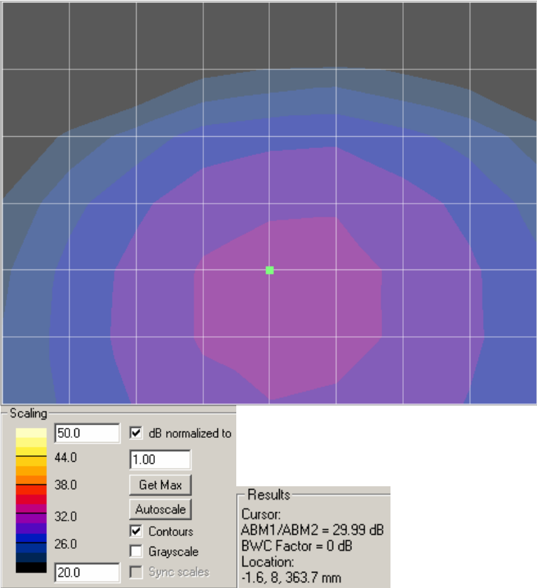
Radial 2 - SNR
