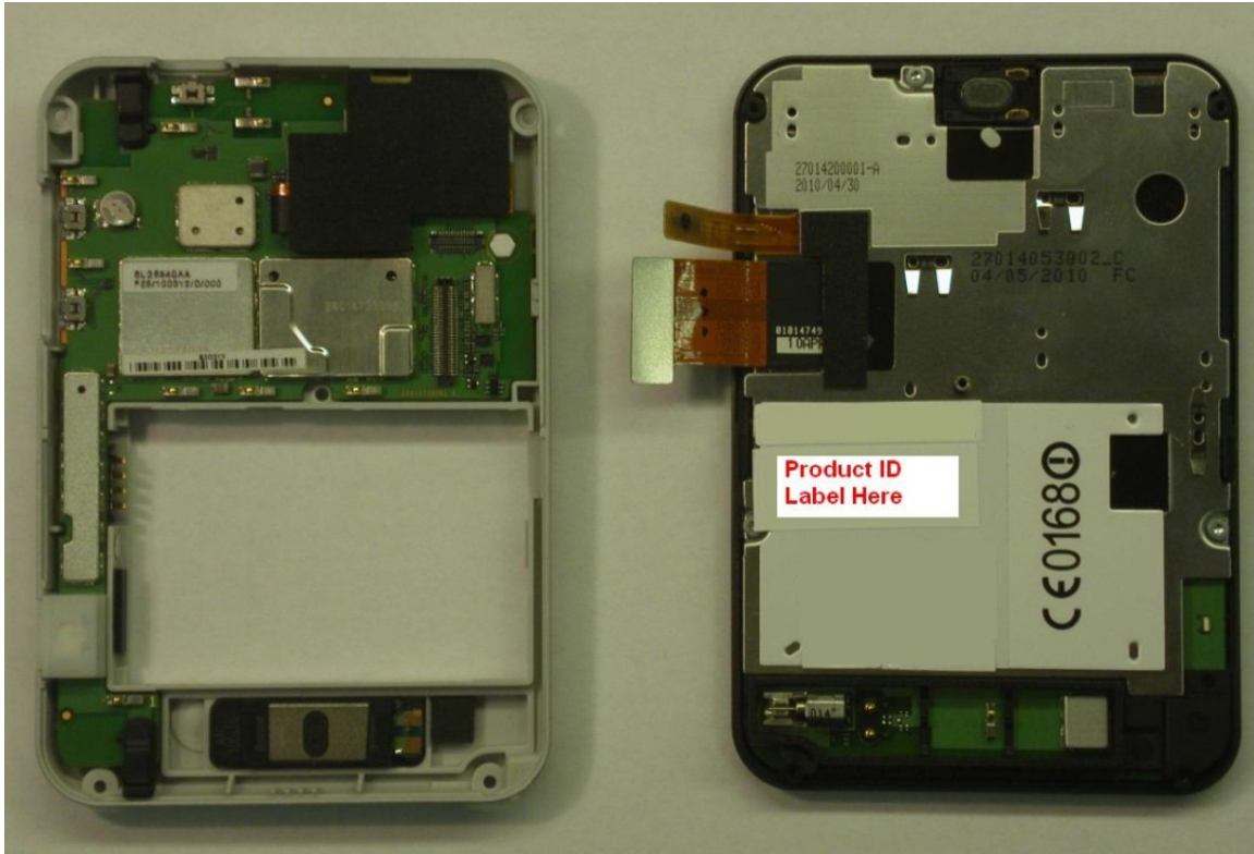
Subassembly Rear
