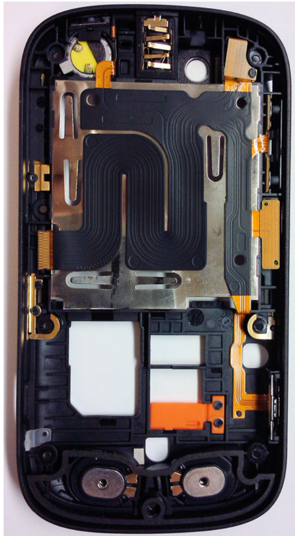
Rear Subassembly
