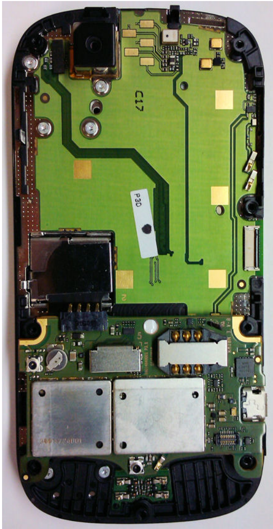
Front Subassembly
