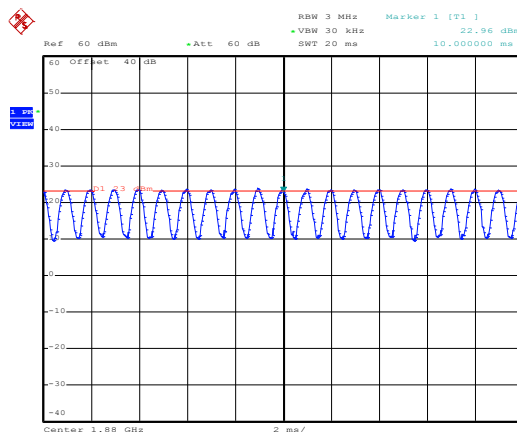
1880MHz - CW
