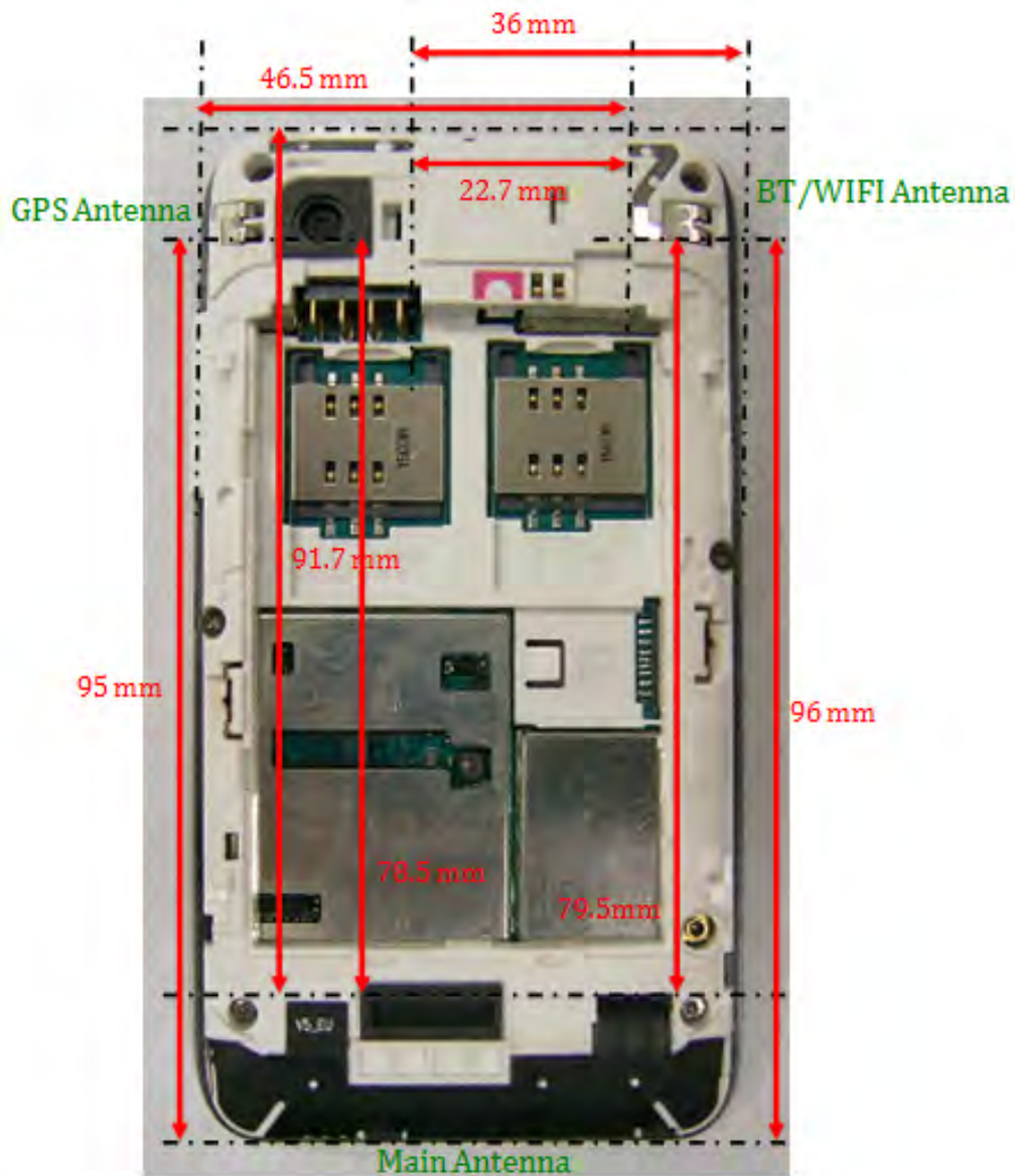
Fig.19 Antenna
