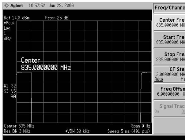
GSM 835 MHz
