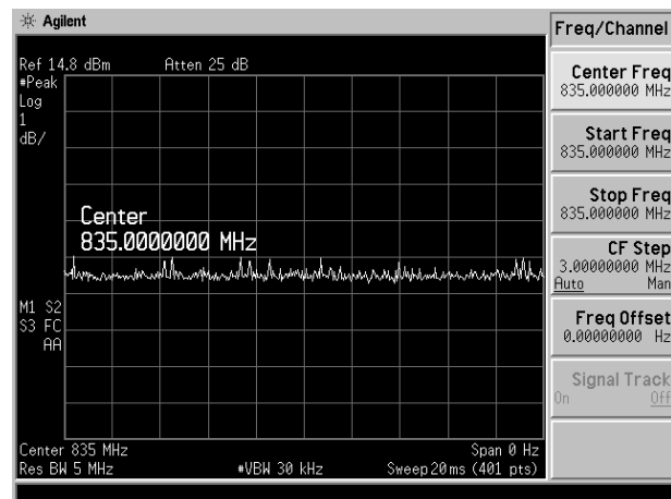
WCDMA 835 MHz
