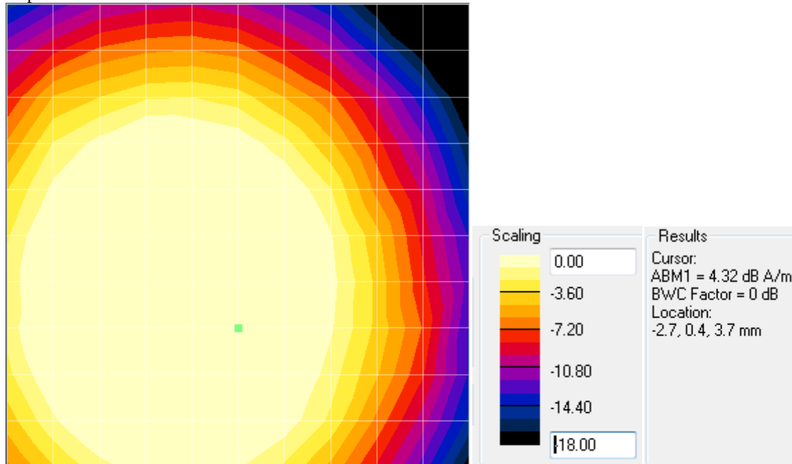
Perpendicular – ABM1
