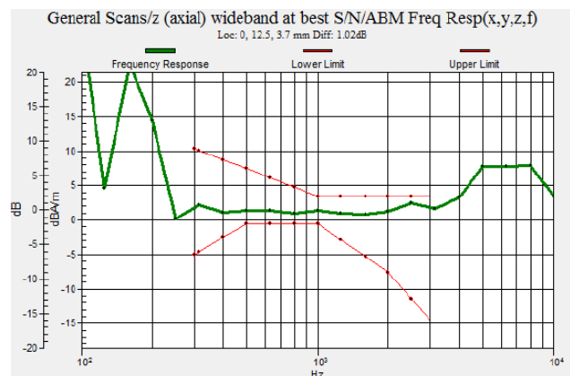
Fig 7.6 CDMA2000 BC10 Ch580
