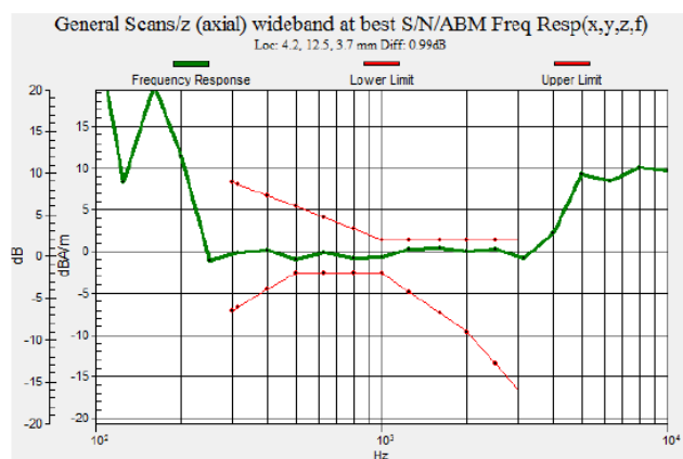
Fig 7.7 CDMA2000 BC1 Ch600
