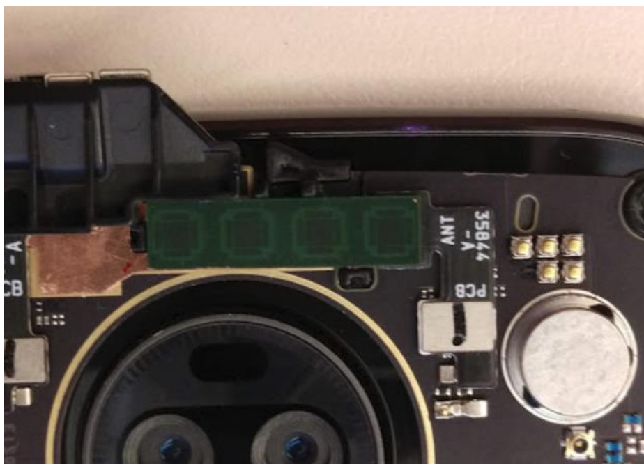
Array Module3
