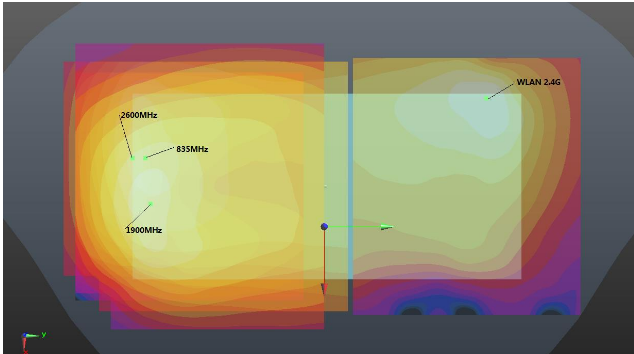
Back(5mm)+WLAN 2.4G(5mm)
