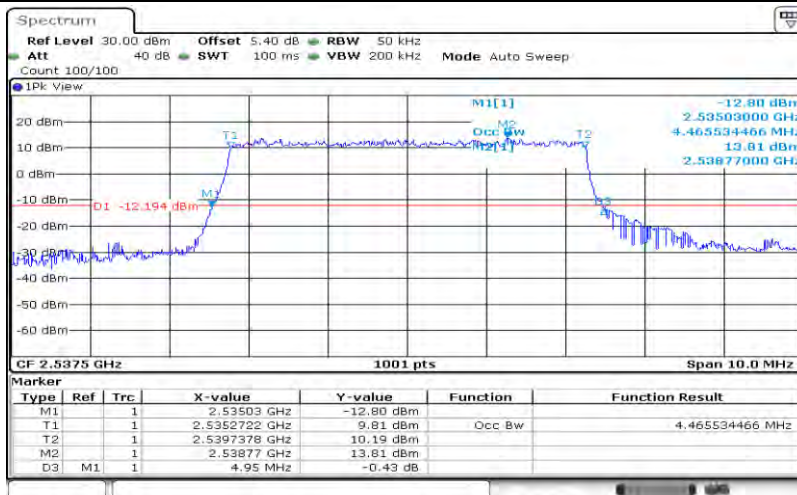
Band41-5MHz-QPSK-40065-25RB#0-4.466
