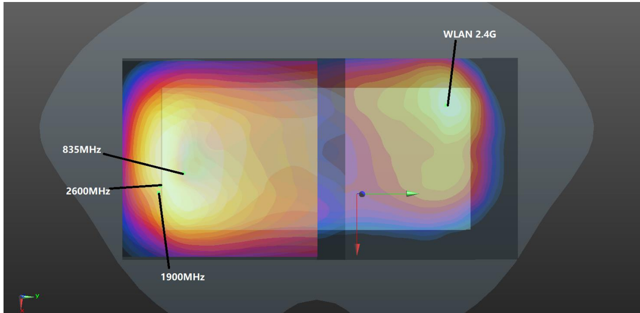
Back(5mm)+WLAN2.4GHz(5mm)
