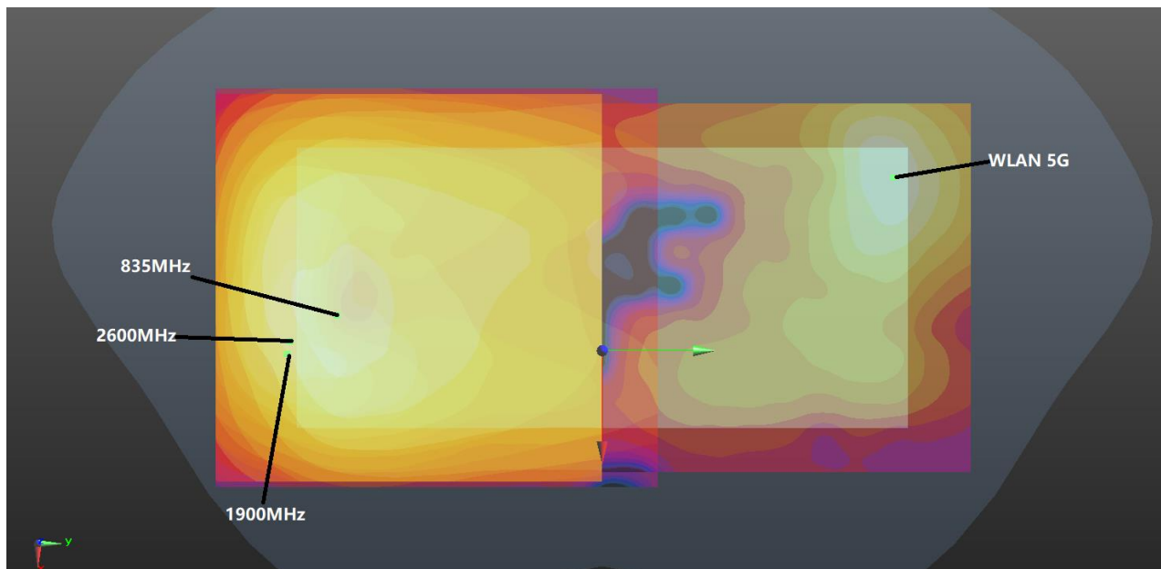
Back(5mm)+WLAN5GHz(5mm)
