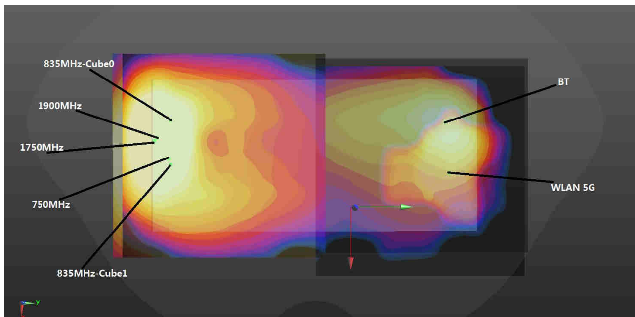
WWAN(5mm)+5GHz(5mm)+BT(5mm)
