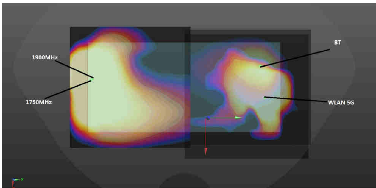
WWAN(23mm)+5GHz(23mm)+BT(23mm)
