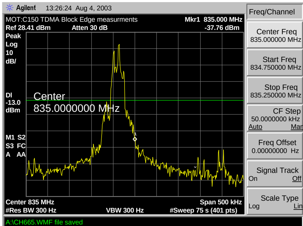
Block A Max Edge/Block B Min.
