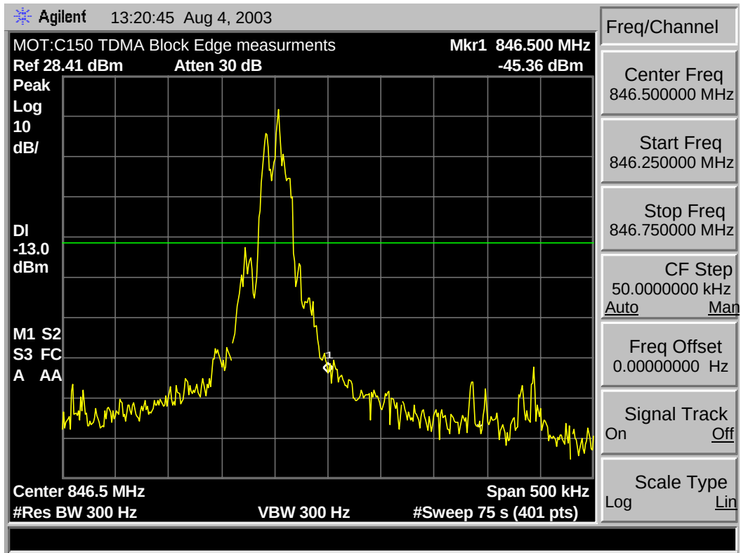
Block A* (Upper) Max Edge/B* Min. Edge
