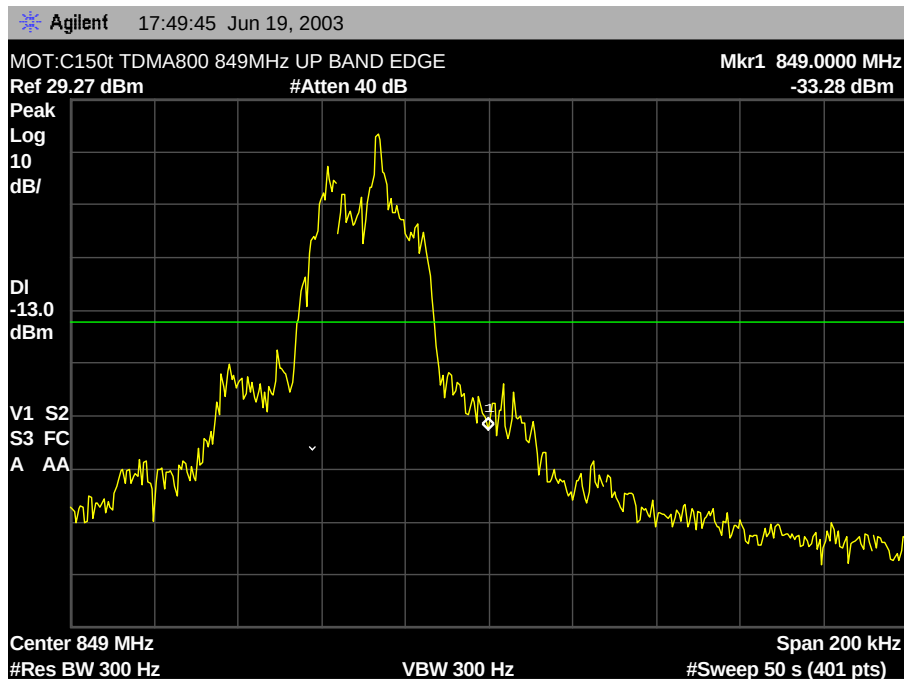
TDMA 800 Upper Band Edge
