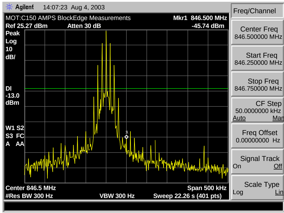
Block A* Upper Max Edge/B* Min.
