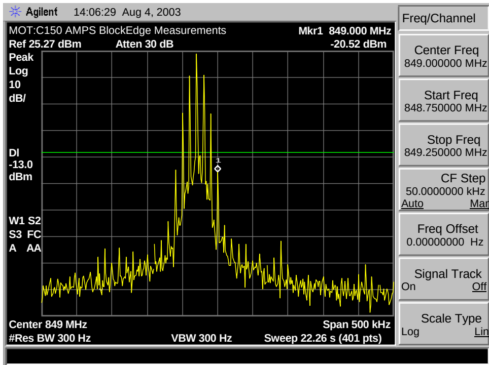
Block B* Max Edge
