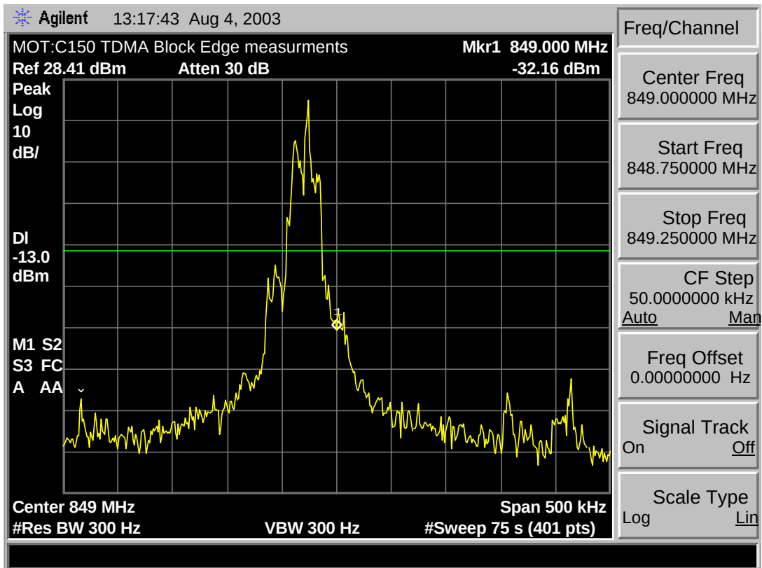
Block B* Max Edge
