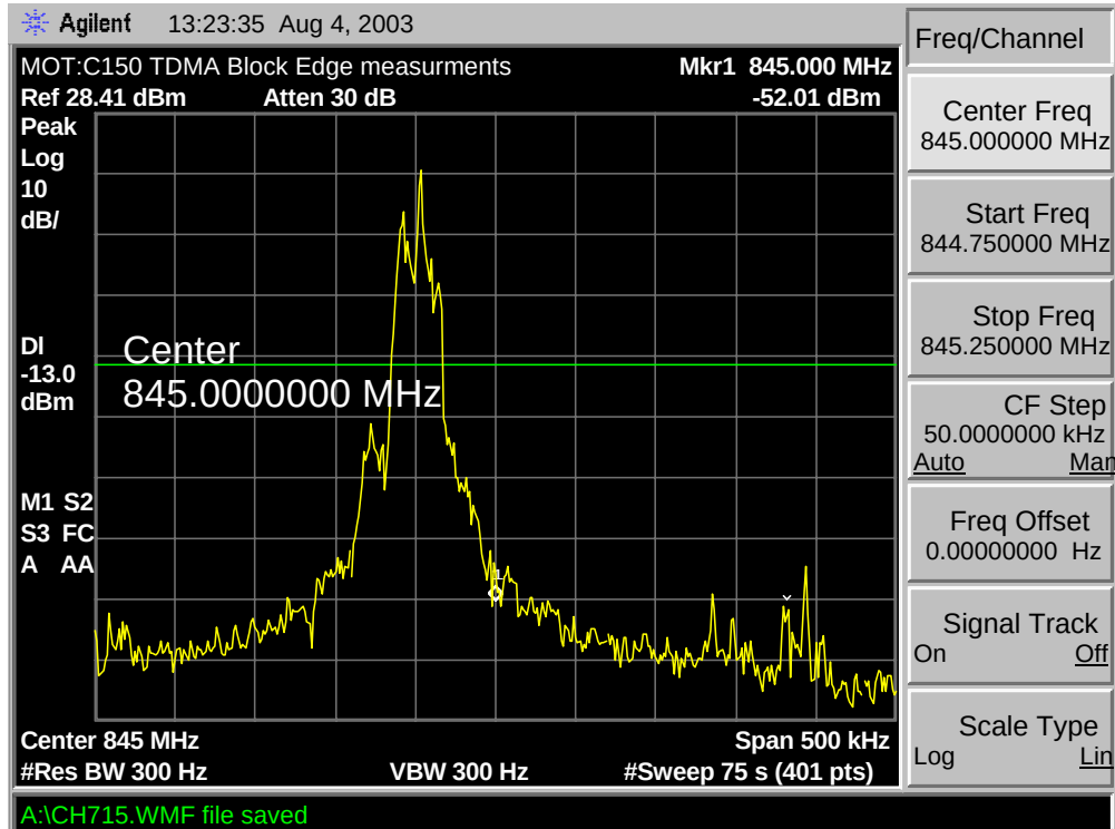
Block B Max Edge/Block A* (Upper) Min. Edge
