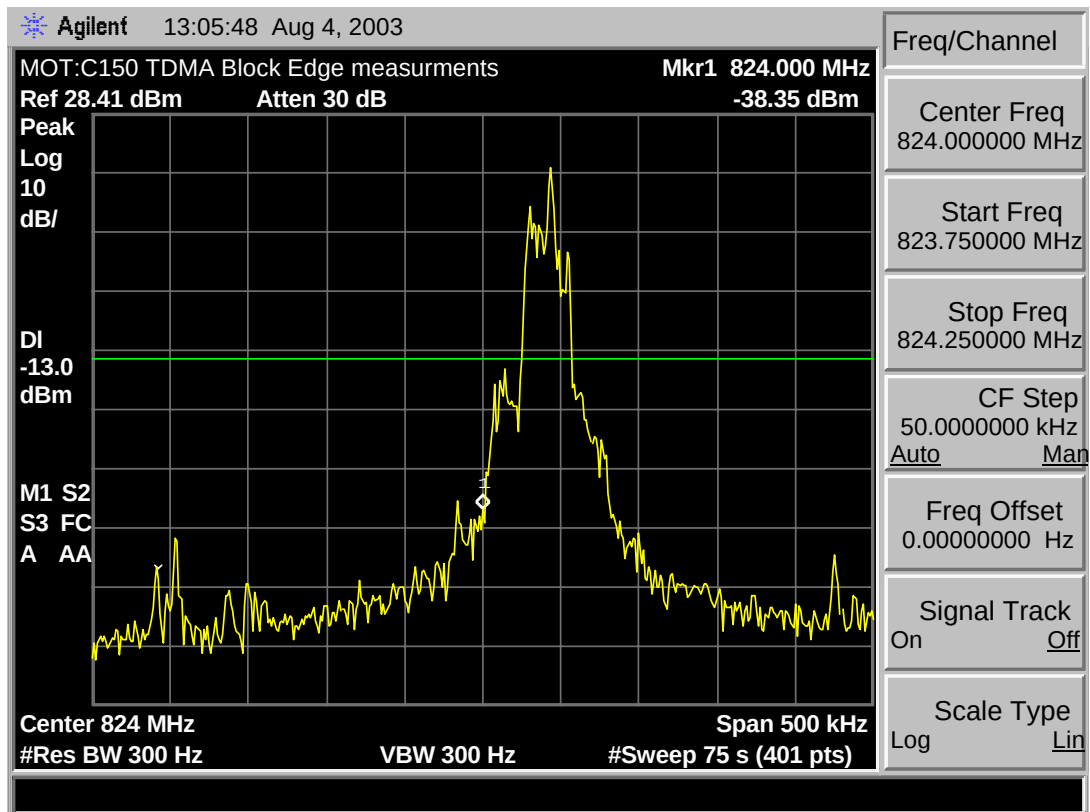
BlockA/A* (Lower) Min. Edge
